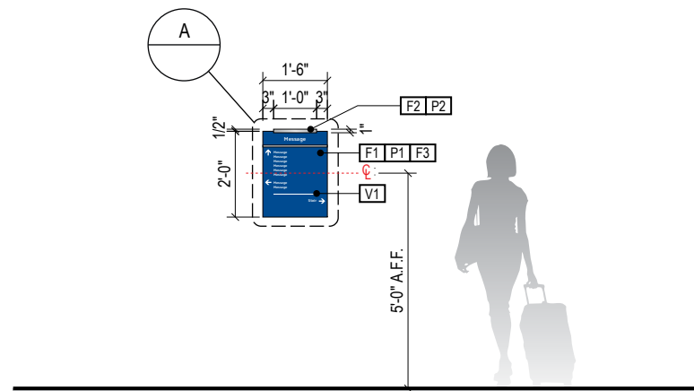
2 ELEVATION Scale: 1/4" = 1'-0"
