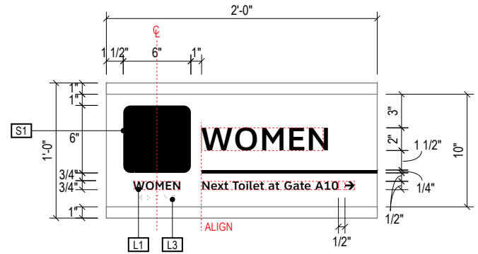
B DETAIL A: Face Layout Scale: 1/2" = 1'-0"
