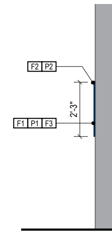
3 END VIEW Scale: 1/4" = 1'-0"
