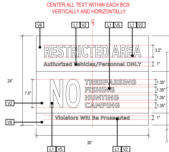
A DETAIL A: Face Layout Scale: NTS
