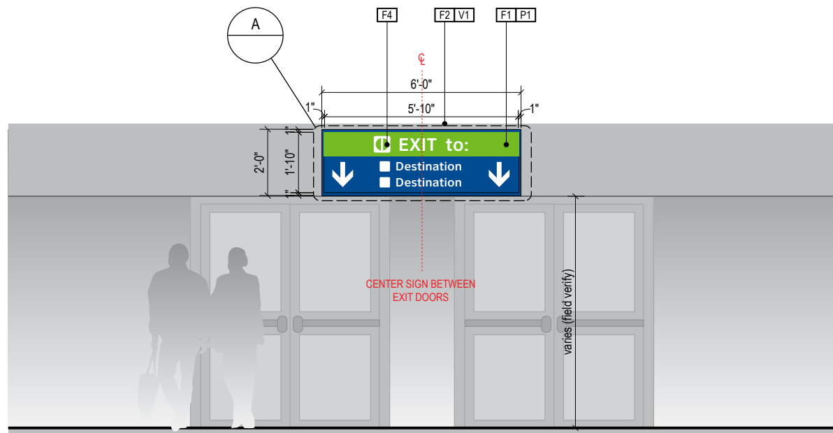
2 ELEVATION Scale: 1/4" = 1'-0"
