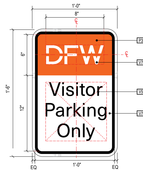
A FACE LAYOUT Scale: NTS
