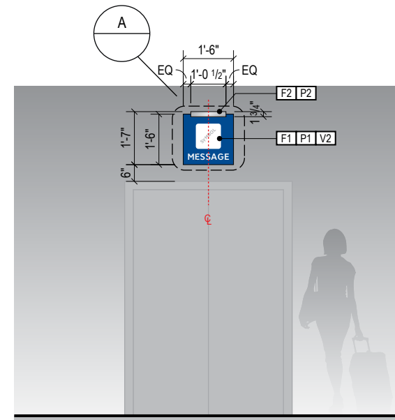
2 ELEVATION Scale: 1/4" = 1'-0"
