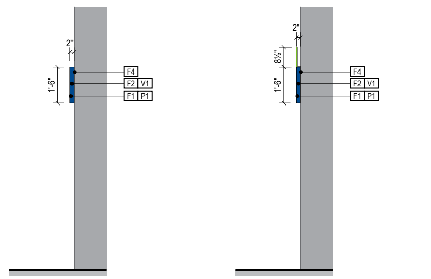
A DETAIL A: Face Layout Scale: 1/4" = 1'-0"
