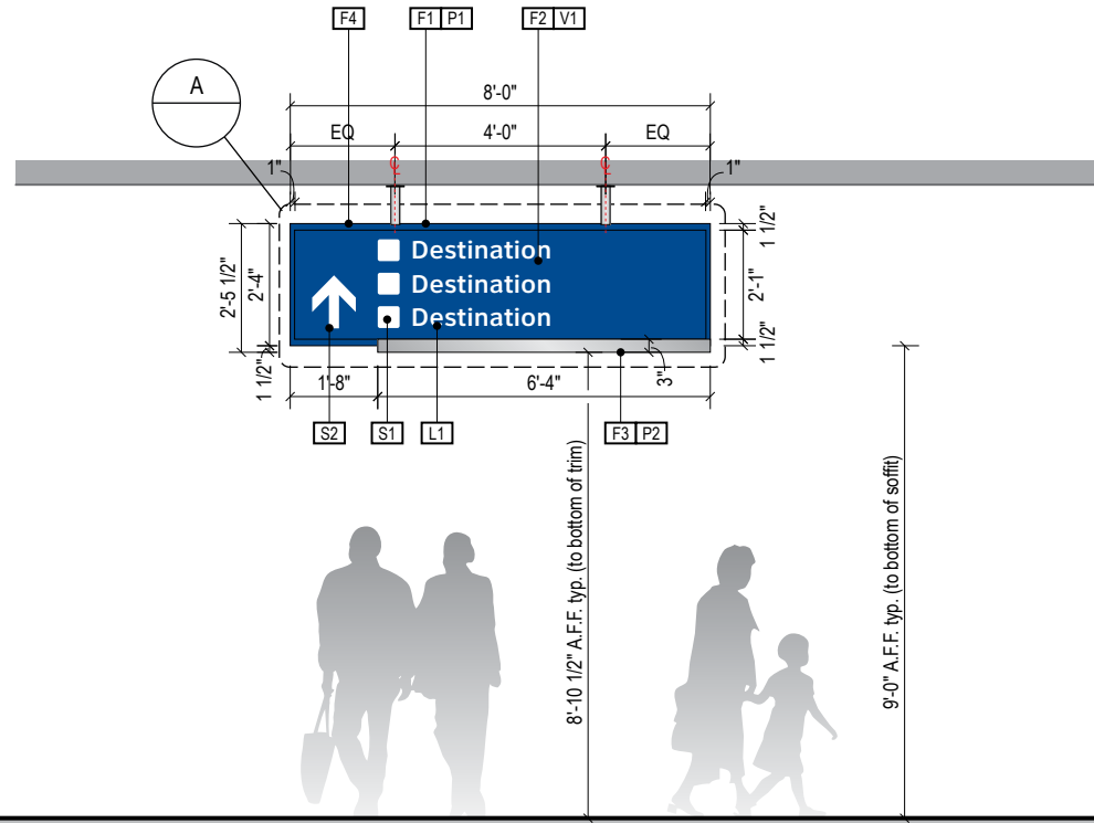
2 ELEVATION Scale: 1/4" = 1'-0"
