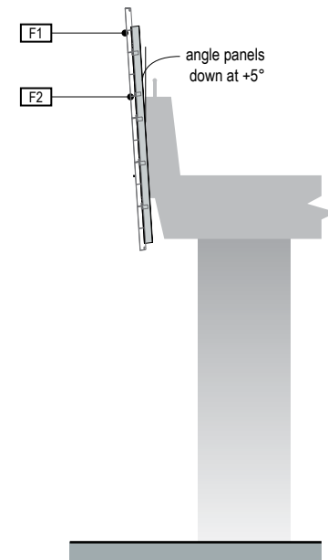
3 ELEVATION Scale: 1/8" = 1'-0"
