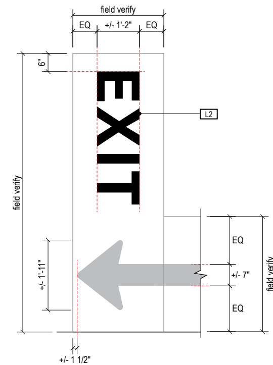
A FACE LAYOUT Scale: 3/8" = 1'-0"
