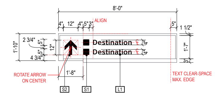
A DETAIL A: Face Layout Scale: 1/4" = 1'-0"
