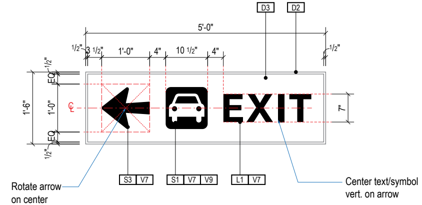
A FACE LAYOUT Scale: 1/2" = 1'-0"
