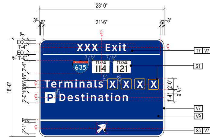
A3 FACE LAYOUT: 4-DR.35 Scale: 3/32" = 1'-0"
