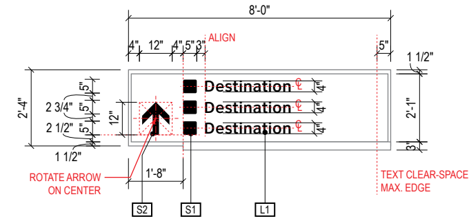
A DETAIL A: Face Layout Scale: 1/4" = 1'-0"
