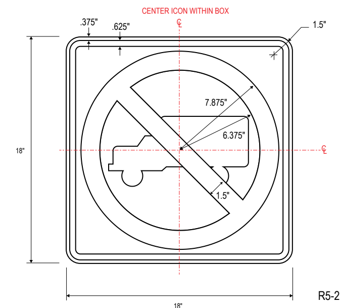
A FACE LAYOUT Alternate Message Scale: NTS
