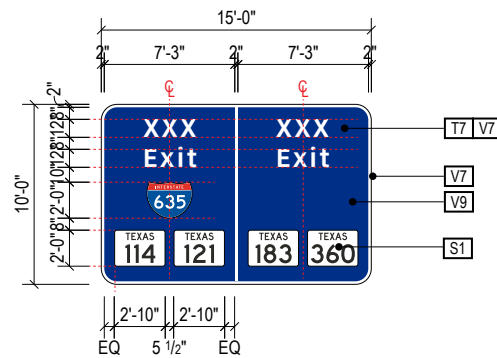
A1 FACE LAYOUT: 4-DR.30 Scale: 3/32" = 1'-0"
