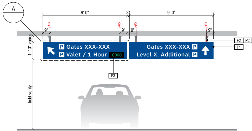
2 ELEVATION Scale: 3/16" = 1'-0"
