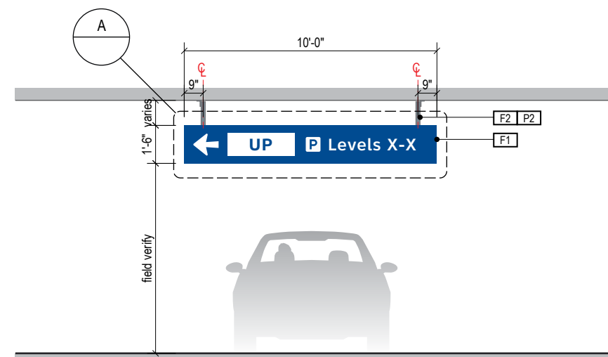
2 ELEVATION Scale: 3/16" = 1'-0"
