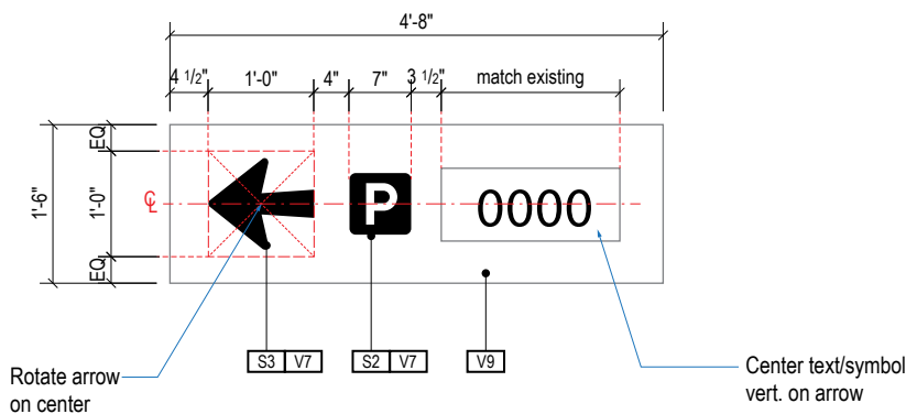
A FACE LAYOUT Scale: 1/2" = 1'-0"
