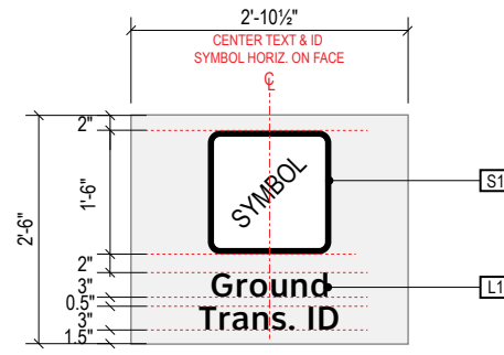
A DETAIL A: Side Face Layout Scale: NTS
