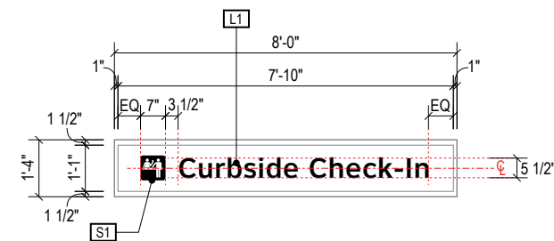
A DETAIL A: Face Layout Scale: 1/4" = 1'-0"
