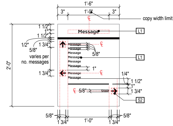
A DETAIL A: Face Layout Scale: 3/4" = 1'-0"
