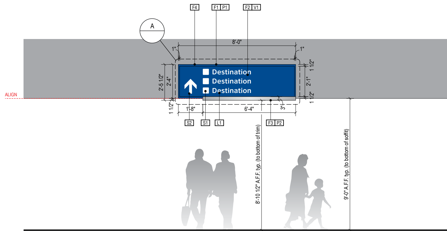
2 ELEVATION Scale: 1/4" = 1'-0"
