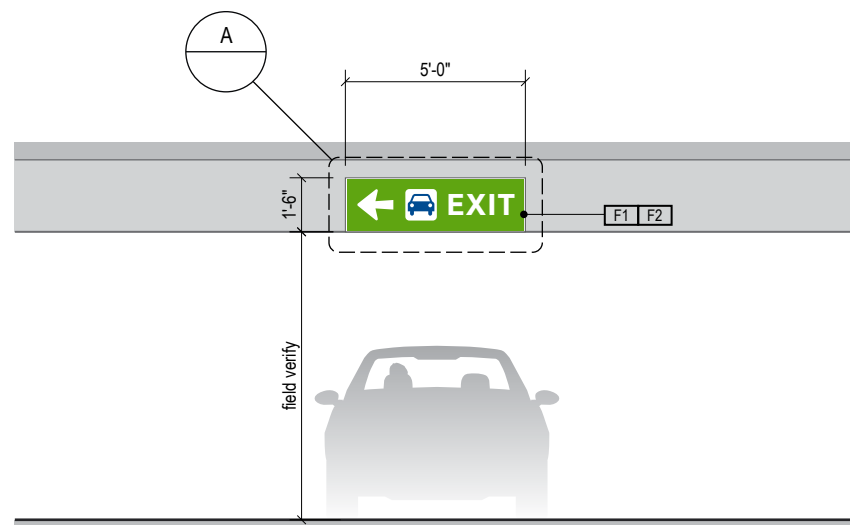
2 ELEVATION Scale: 3/16" = 1'-0"
