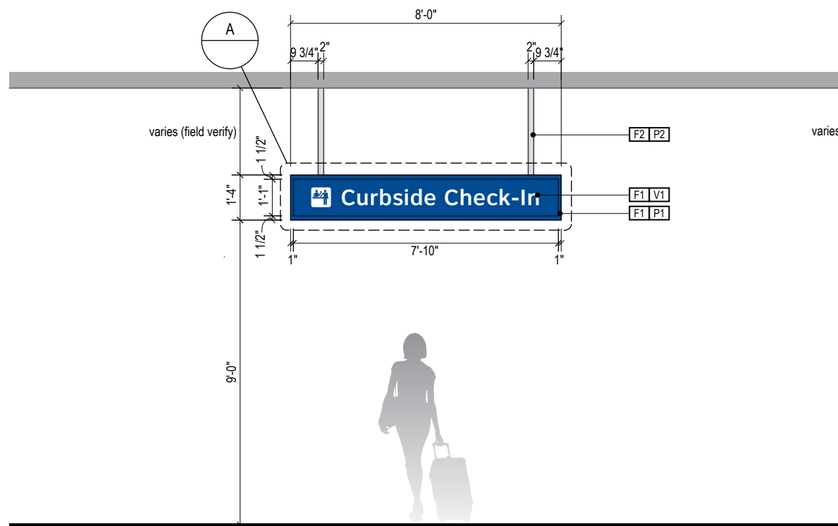
2 ELEVATION Scale: 1/4" = 1'-0"
