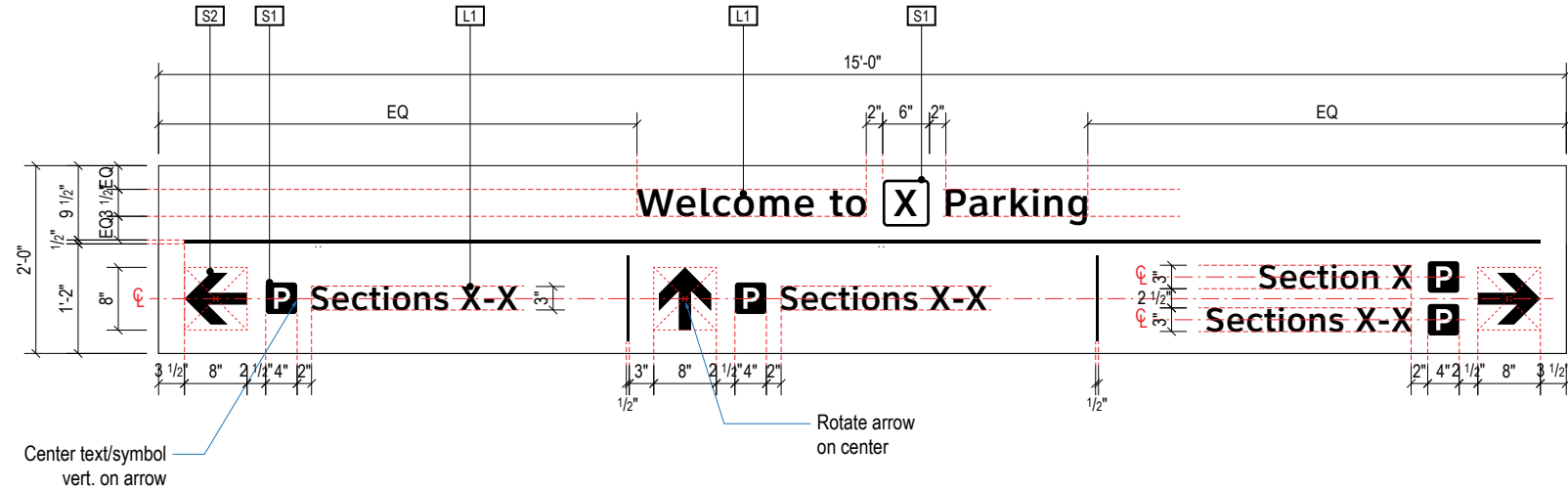
A FACE LAYOUT Scale: 1/2" = 1'-0"
