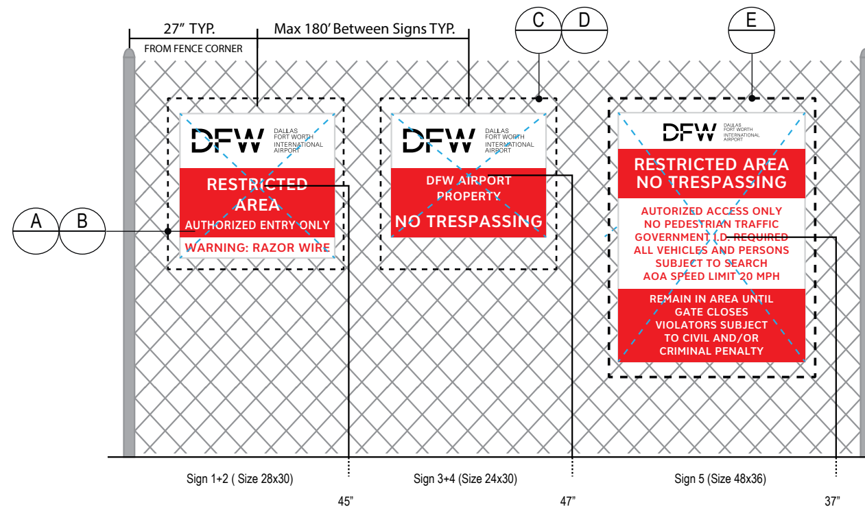
2 ELEVATION
