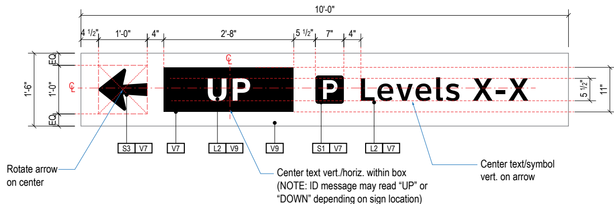
A FACE LAYOUT Scale: 1/2" = 1'-0"
