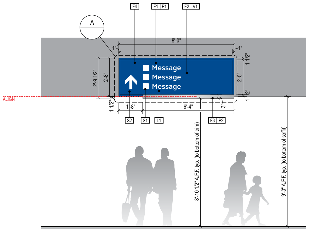
2 ELEVATION Scale: 1/4" = 1'-0"
