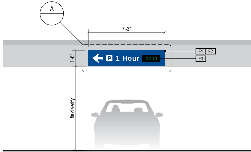
2 ELEVATION Scale: 3/16" = 1'-0"
