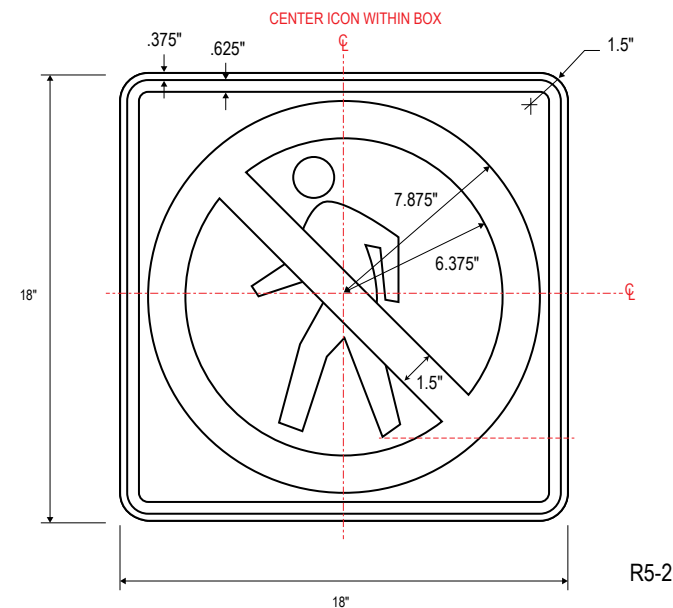
A FACE LAYOUT Scale: NTS
