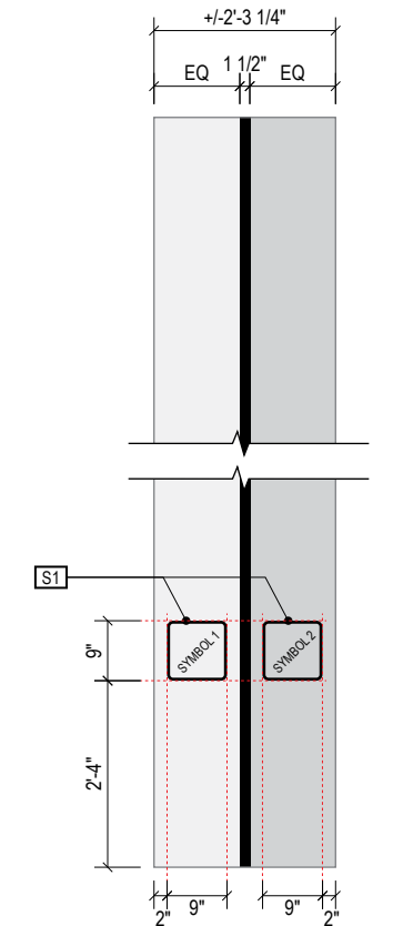
B DETAIL B: Face Layout Scale: 3/8" = 1'-0"
