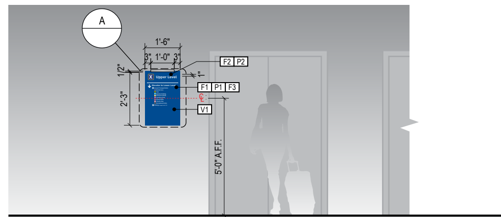
2 ELEVATION Scale: 1/4" = 1'-0"
