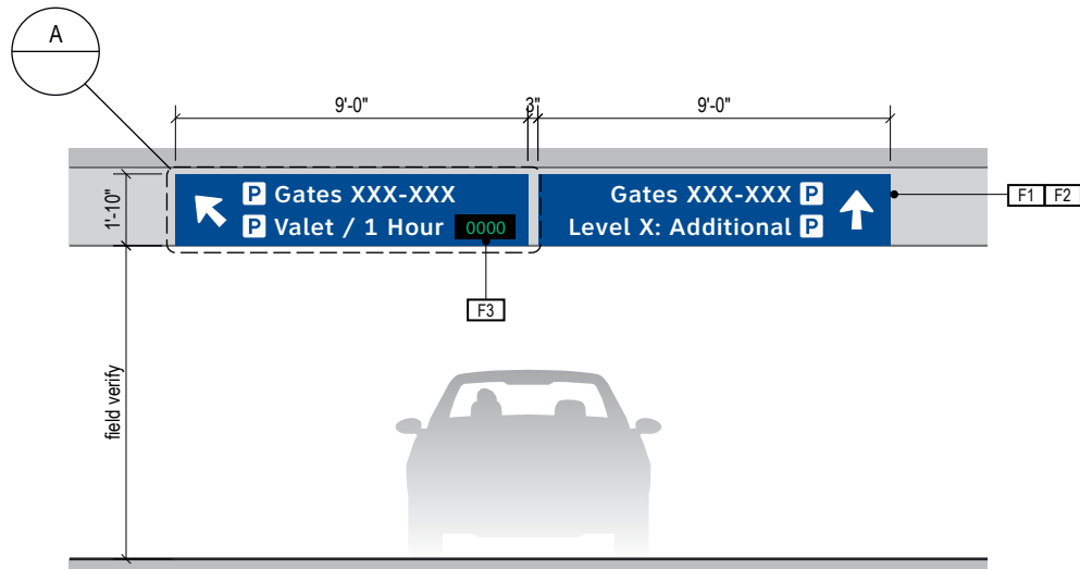
2 ELEVATION Scale: 3/16" = 1'-0"
