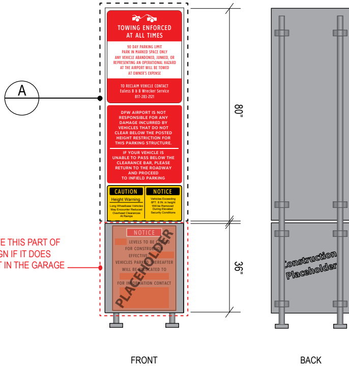
2 ELEVATION Scale: NTS
