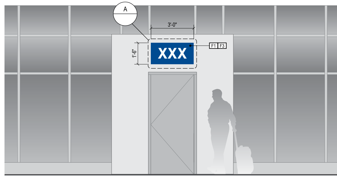
2 ELEVATION Scale: 1/4" = 1'-0"
