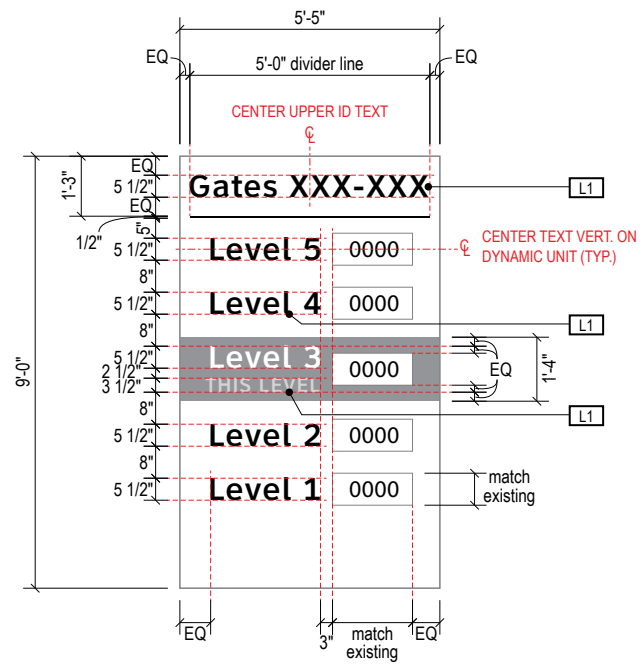
A FACE LAYOUT Scale: 1/4" = 1'-0"
