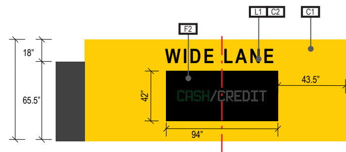
A FACE LAYOUT Scale: NTS
