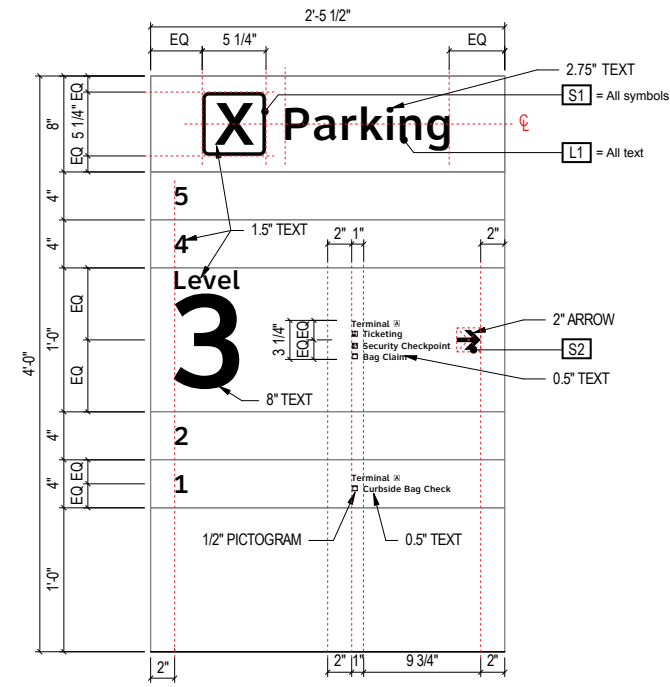
A DETAIL A: Face Layout Scale: 3/4" = 1'-0"
