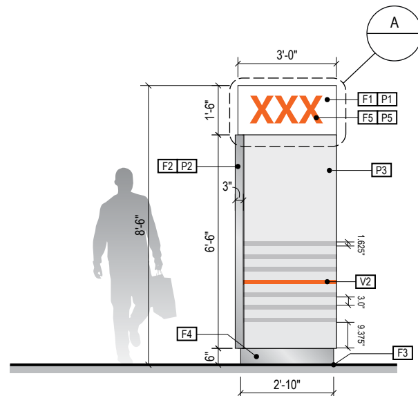
2 ELEVATION Scale: 1/4" = 1'-0"
