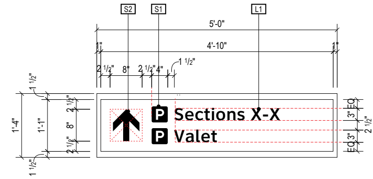
B FACE LAYOUT Scale: 1/2" = 1'-0"
