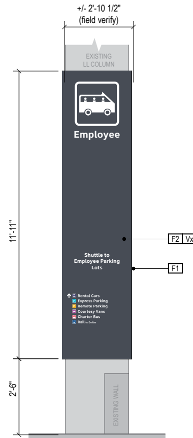
4 RIGHT SIDE Scale: 1/4" = 1'-0"
