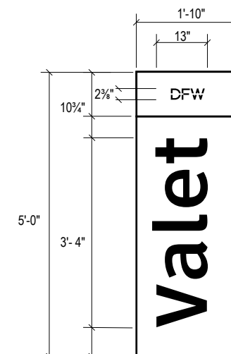
A FACE LAYOUT: Valet Scale: 1/2" = 1'-0"
