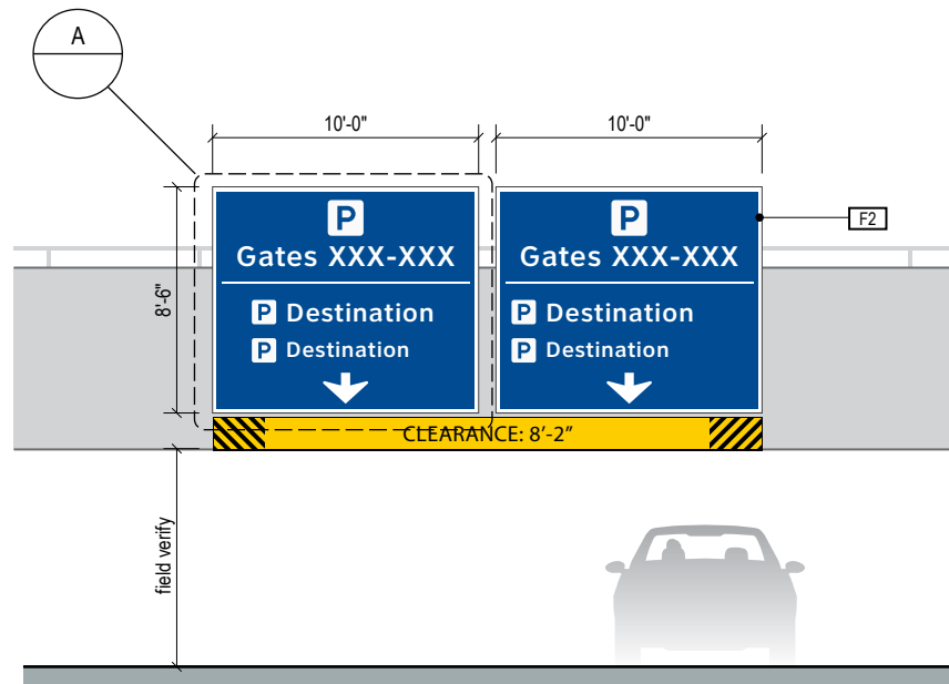
2 ELEVATION Scale: 1/8" = 1'-0"
