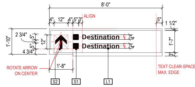
A DETAIL A: Face Layout Scale: 1/4" = 1'-0"
