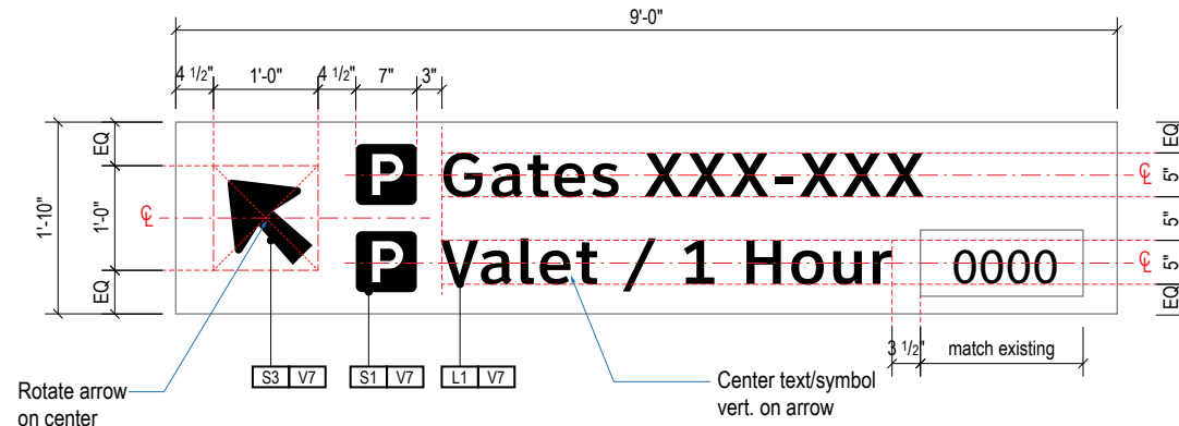
A FACE LAYOUT Scale: 1/2" = 1'-0"
