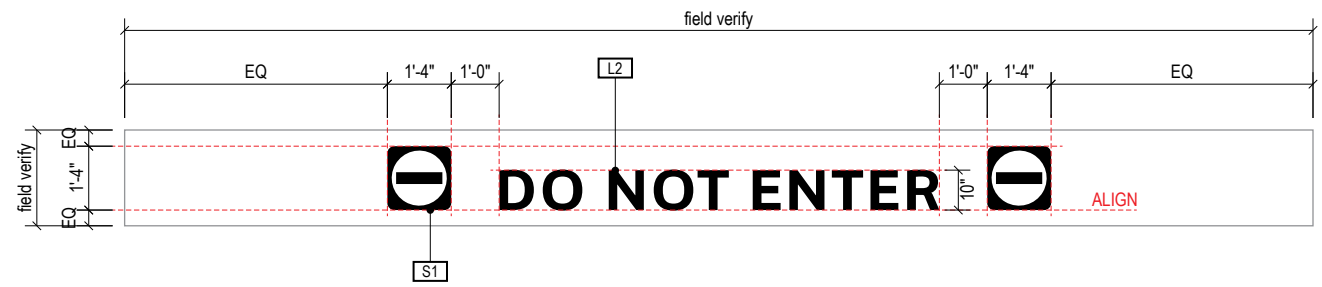
A FACE LAYOUT Scale: 1/4" = 1'-0"
