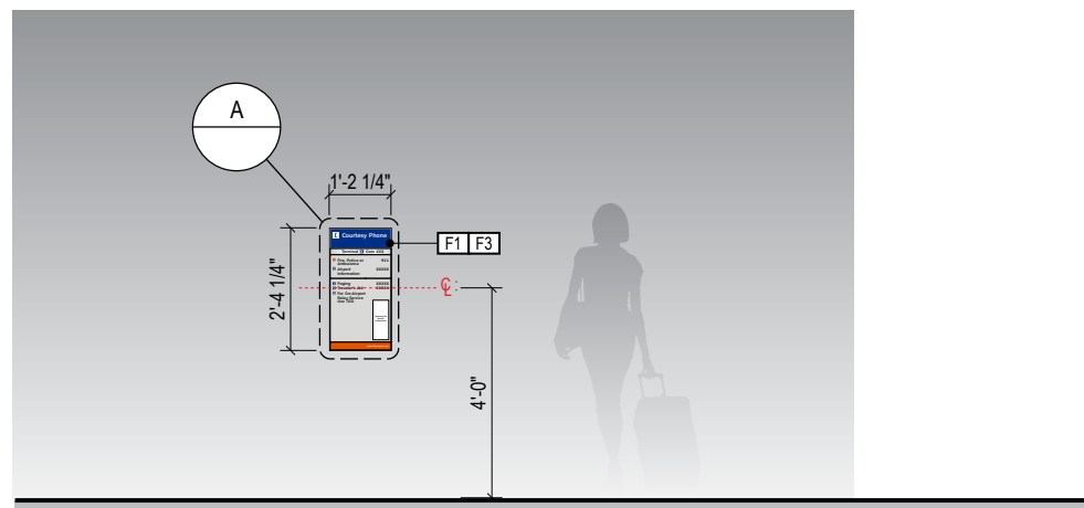
3 ELEVATION
