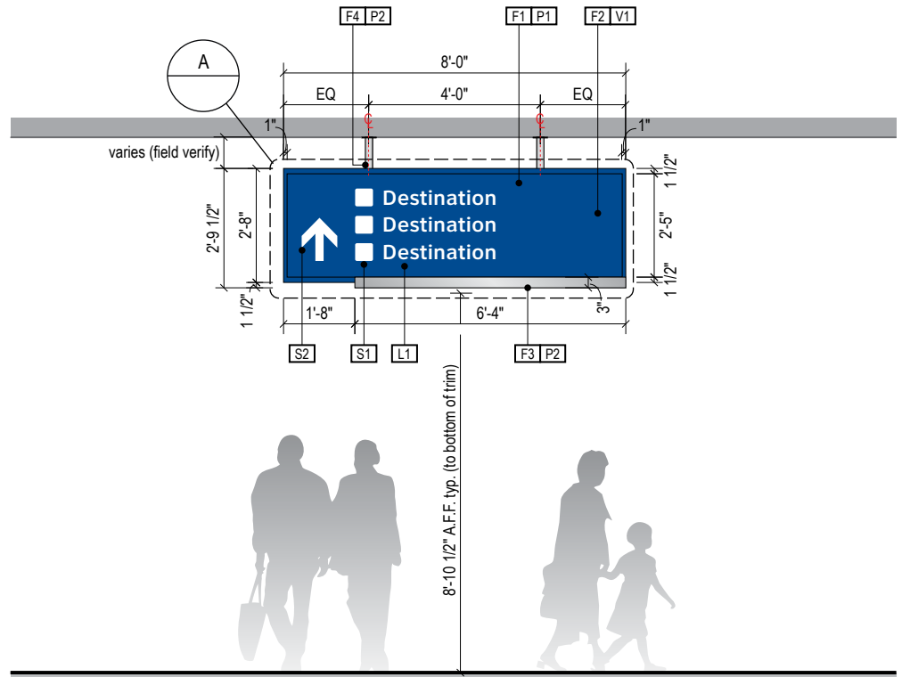
2 ELEVATION
