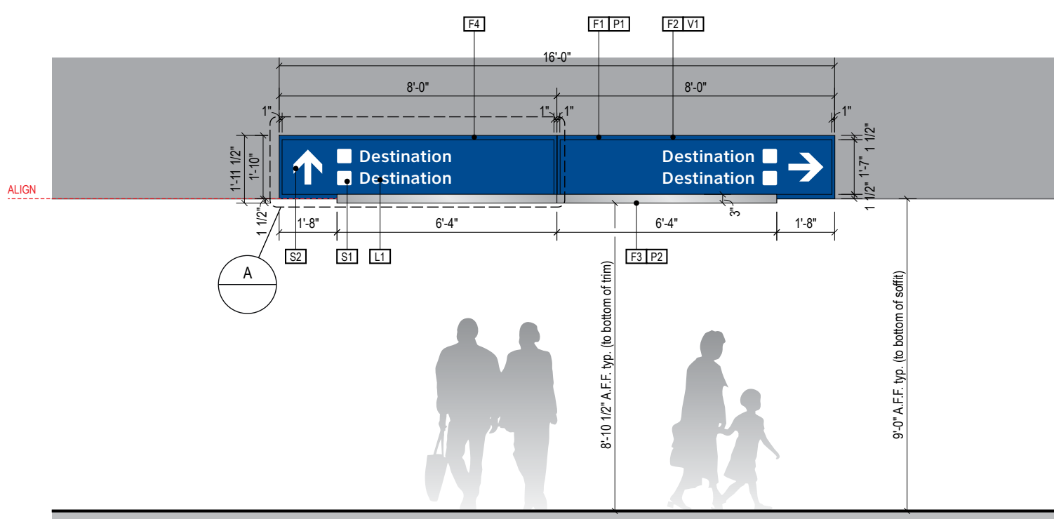
2 ELEVATION Scale: 1/4" = 1'-0"
