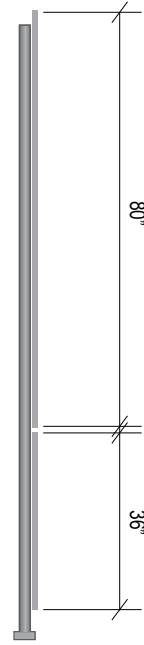
3 END VIEW Scale: NTS
