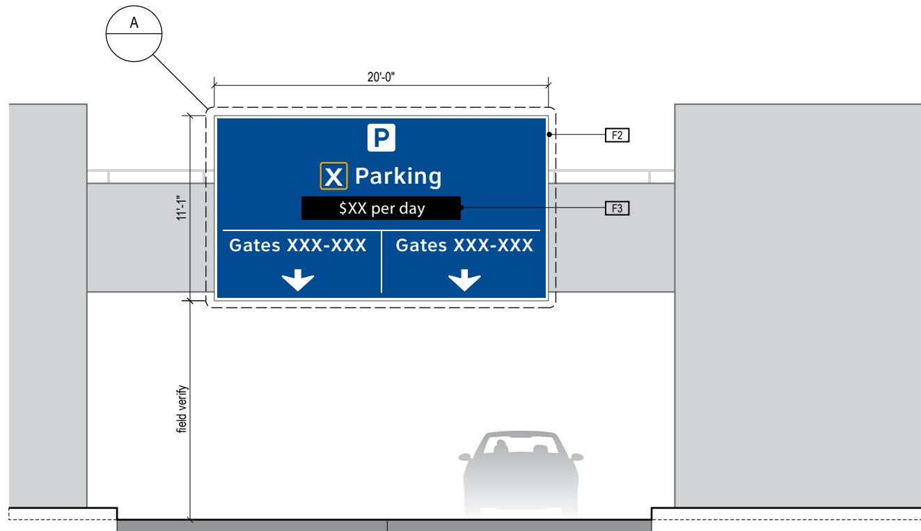
2 ELEVATION Scale: 1/8" = 1'-0"
