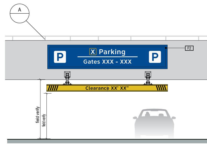
2 ELEVATION Scale: 1/8" = 1'-0"
