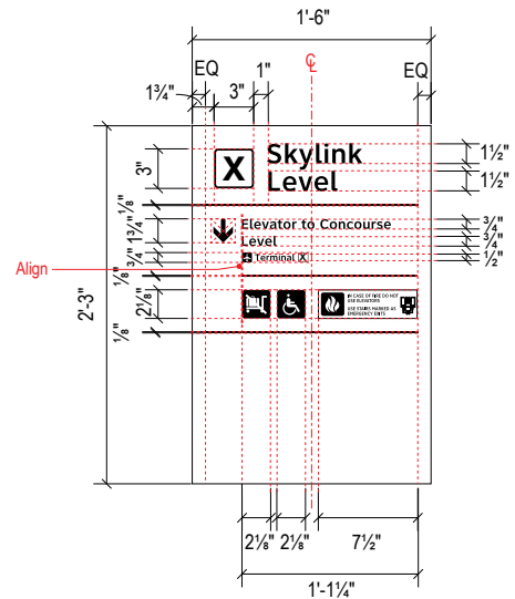
A DETAIL A: Face Layout Scale: 3/4" = 1'-0"
