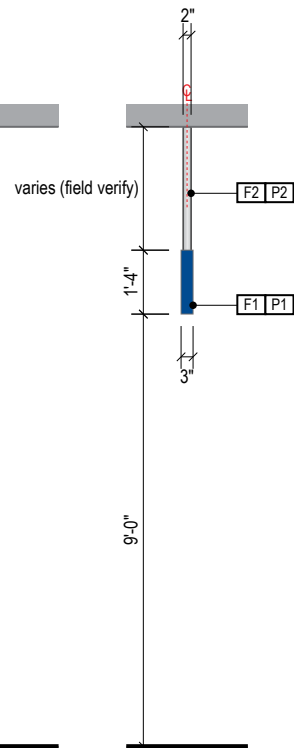
3 END VIEW Scale: 1/4" = 1'-0"
