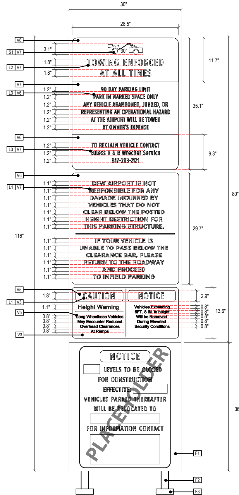
A FACE LAYOUT Scale: NTS
