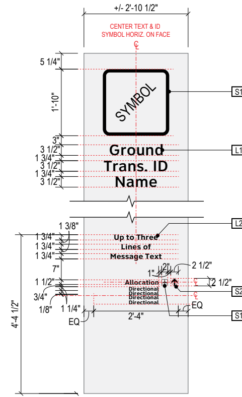
A DETAIL A: Face Layout Scale: 3/8" = 1'-0"
