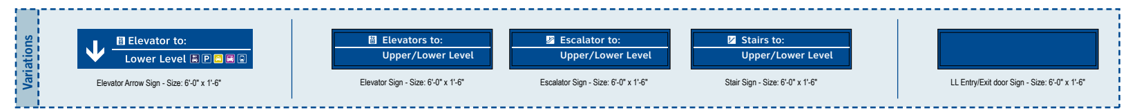
A DETAIL A: Face Layout Scale: 1/4" = 1'-0"
