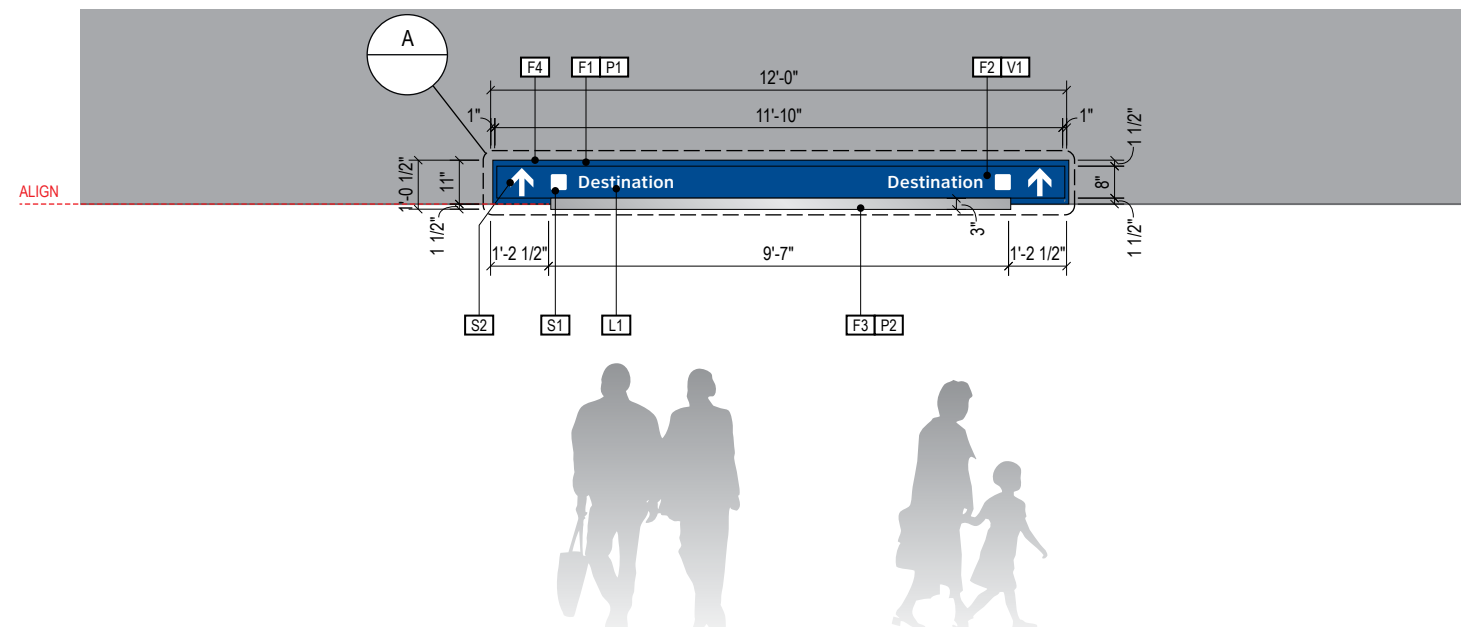
2 ELEVATION Scale: 1/4" = 1'-0"
