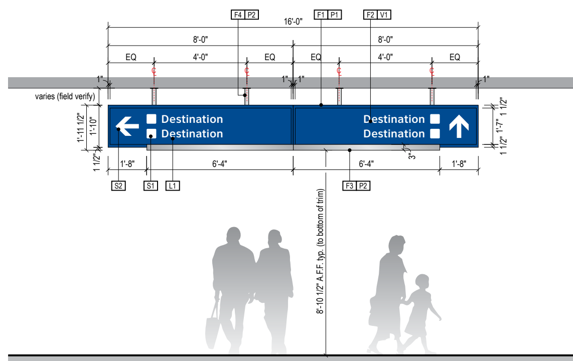
2 ELEVATION Scale: 1/4" = 1'-0"
