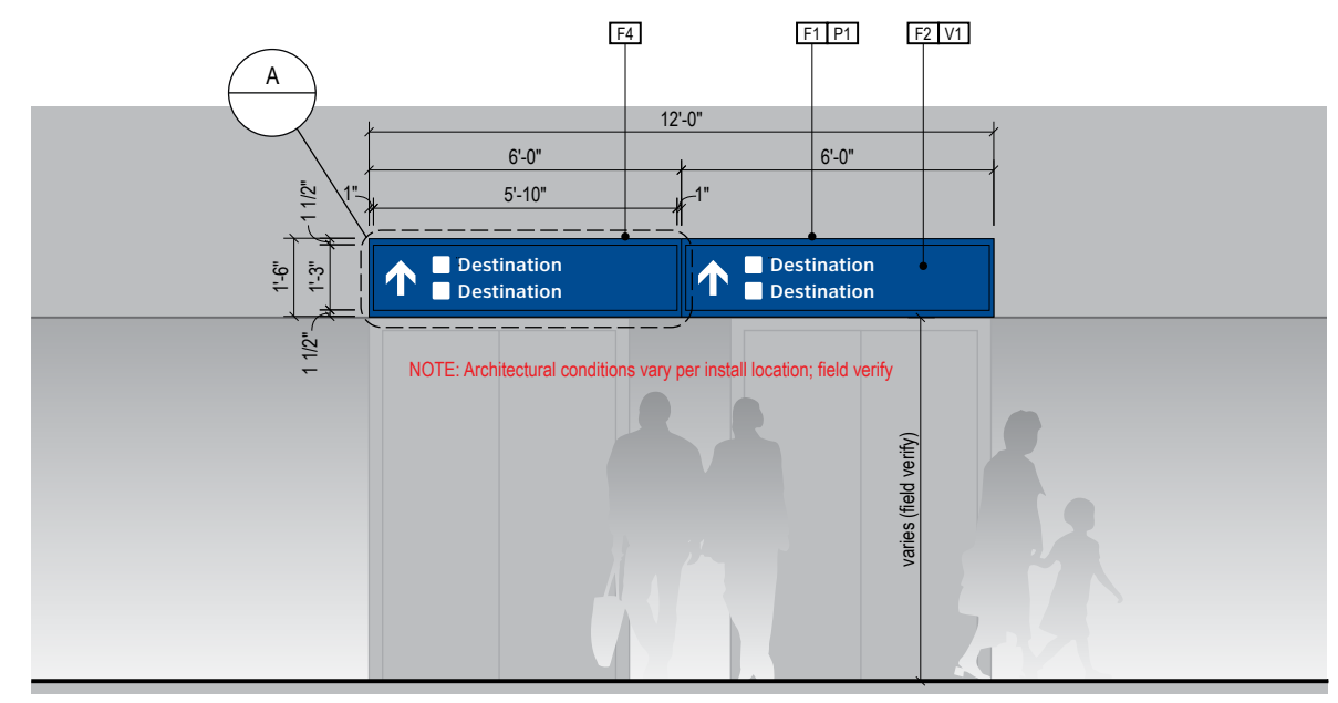
3a ELEVATION ELEVATOR Scale: 1/4" = 1'-0"
