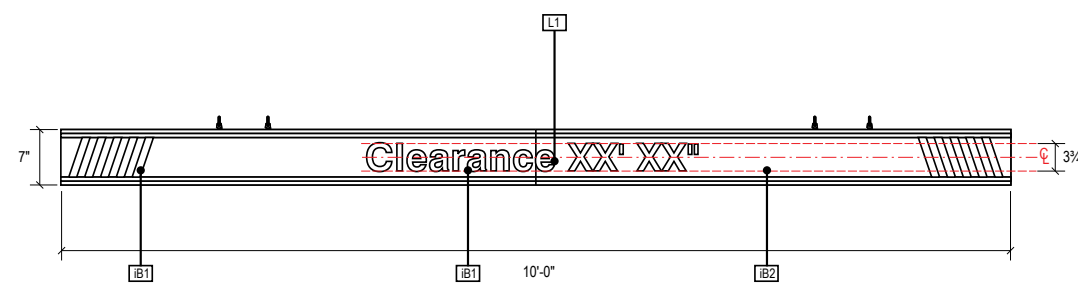
A DETAIL A: FACE LAYOUT Scale: 1/4" = 1'-0"
