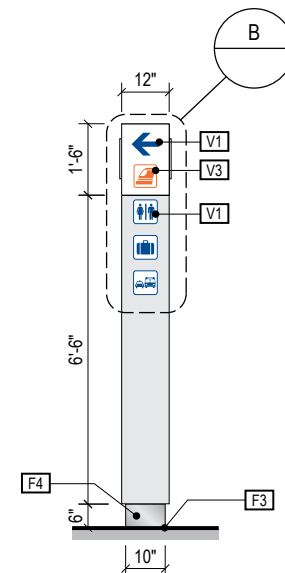
3 END VIEW Scale: 1/4" = 1'-0"
