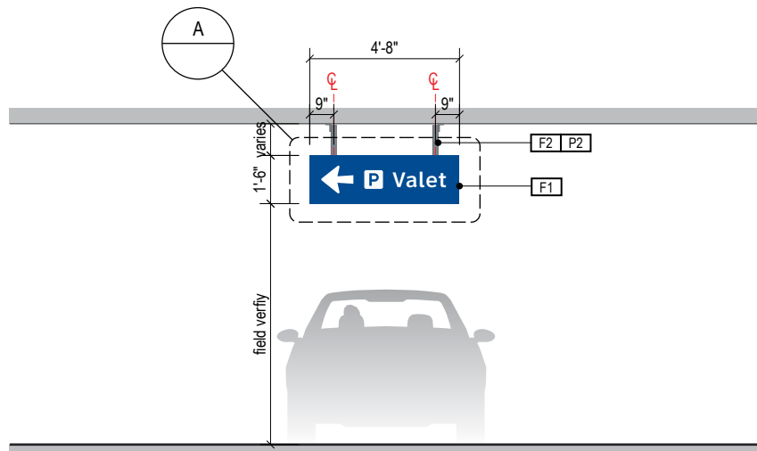
2 ELEVATION Scale: 3/16" = 1'-0"
