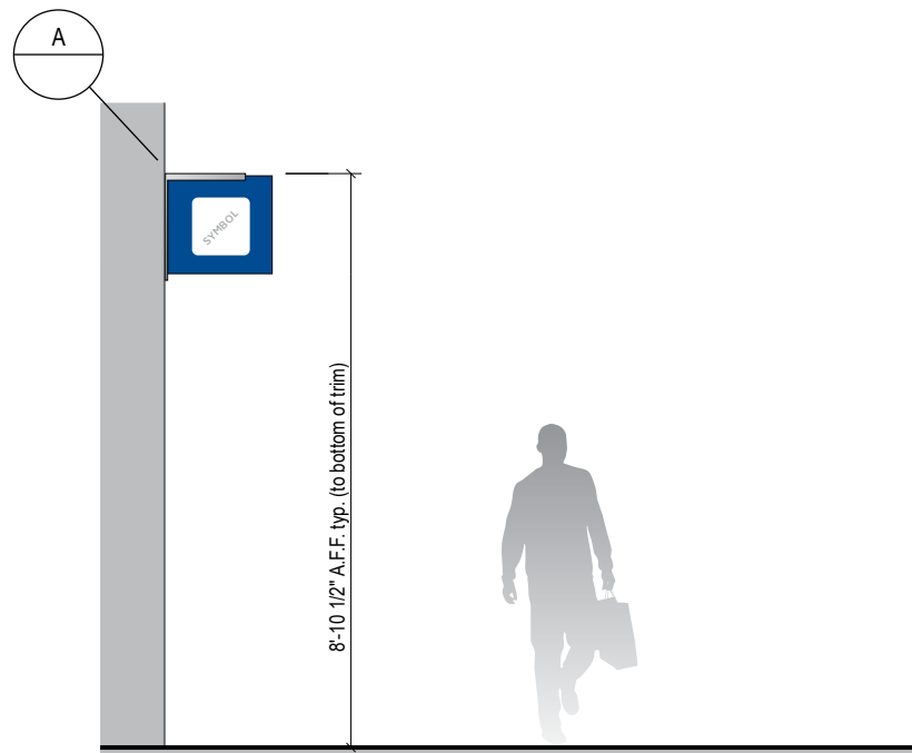
2 ELEVATION Scale: 1/4" = 1'-0"
