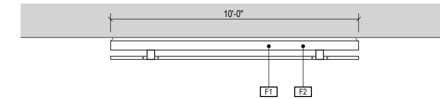
1 PLAN VIEW Scale: 1/8" = 1'-0"
