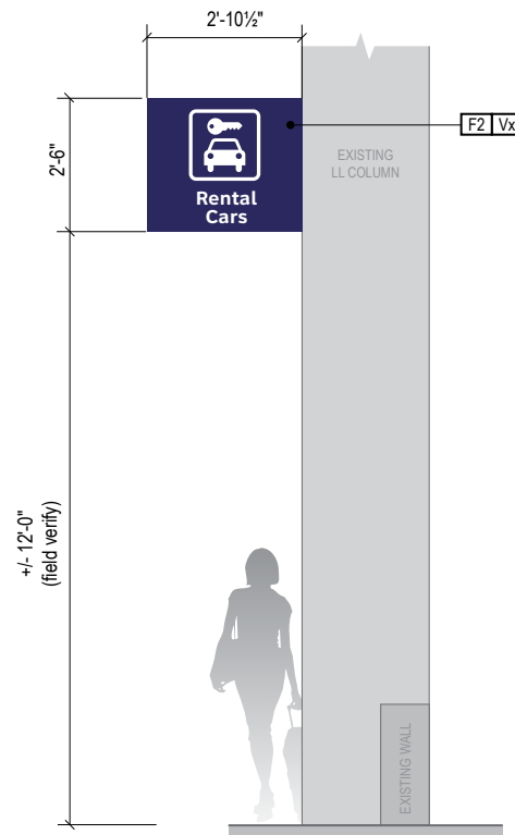
4 RIGHT SIDE Scale: NTS
