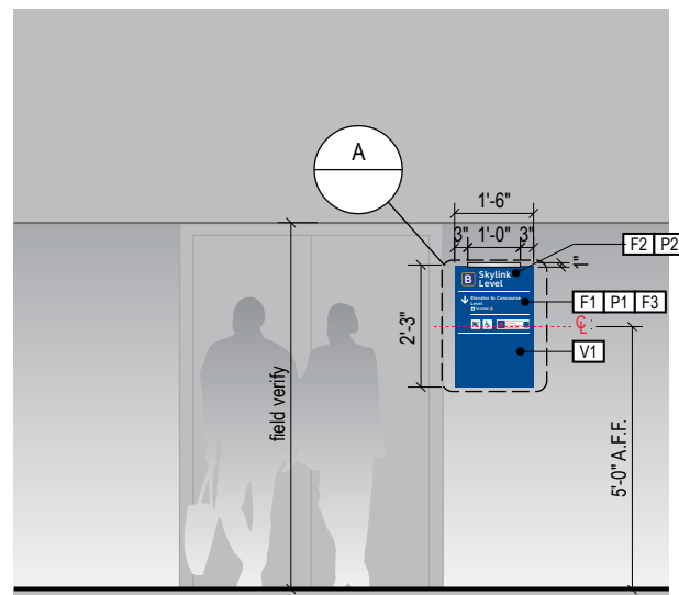
2 ELEVATION Scale: 1/4" = 1'-0"
