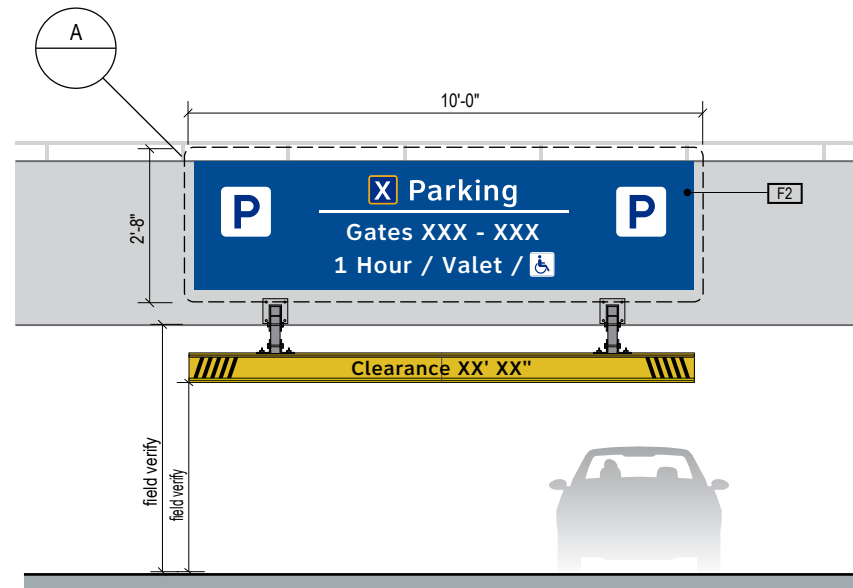
2 ELEVATION Scale: 1/8" = 1'-0"
