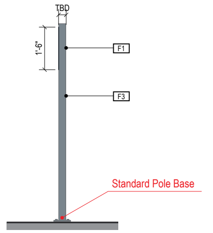
3 END VIEW Scale: NTS
