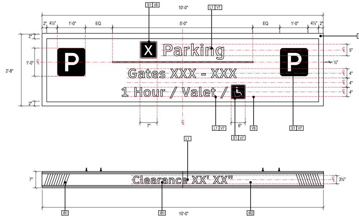
A DETAIL A: FACE LAYOUT Scale: 1/4" = 1'-0"
