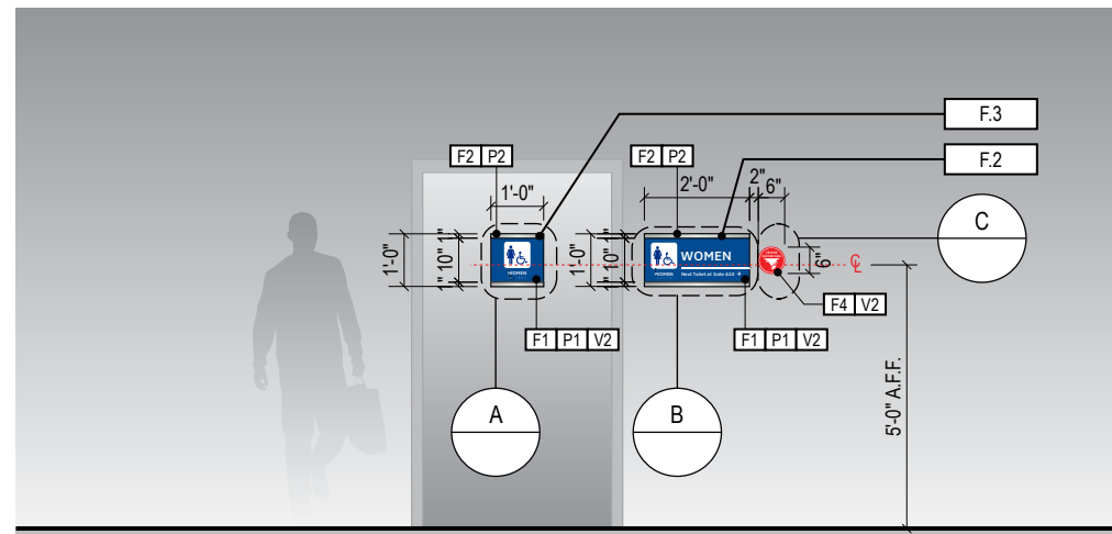
1 ELEVATION Scale: 1/4" = 1'-0"
