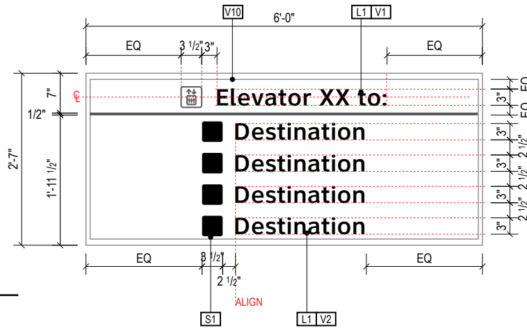
A DETAIL A: Face Layout Scale: 1/2" = 1'-0"
