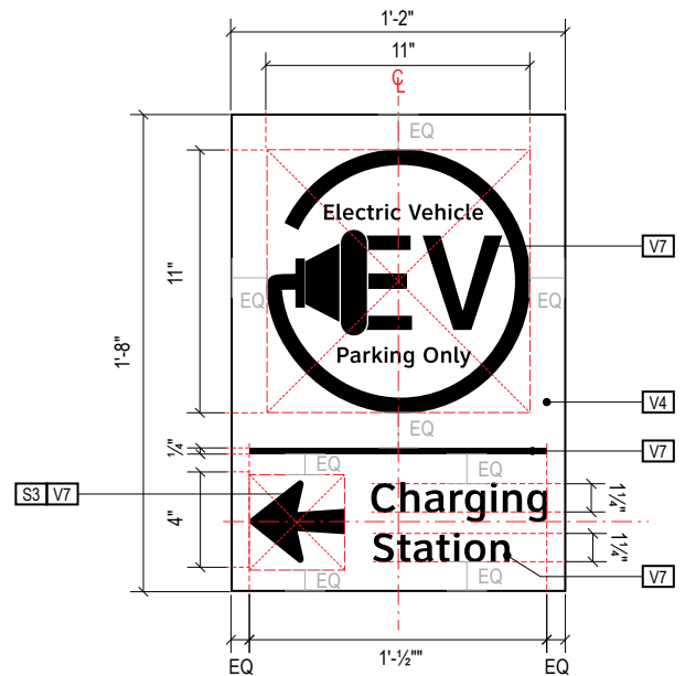
A FACE LAYOUT Scale: NTS
