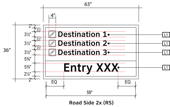
A DETAIL A: FACE LAYOUT Scale: 1/4" = 1'-0"
