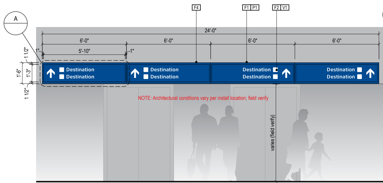
3a ELEVATION ELEVATOR Scale: 1/4" = 1'-0"
