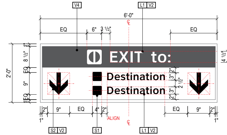
A DETAIL A: Face Layout Scale: 1/2" = 1'-0"
