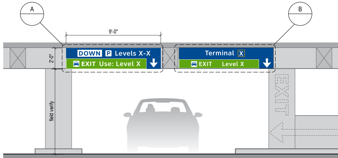
2 ELEVATION Scale: 3/16" = 1'-0"
