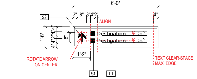
A DETAIL A: Face Layout Scale: 1/4" = 1'-0"
