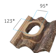
Teja con salida circular
