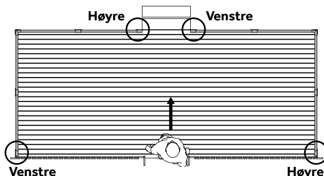
Skisse for plassering av frontmonterte endestolper
