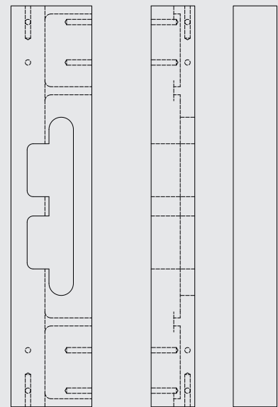
Frässhablone für SB/VAR.ST und SB/VAR.ST/x/LAP5
