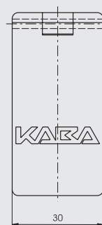
ROS/E/WS/ALU Zeichnung inkl. Unterlagsplättchen
