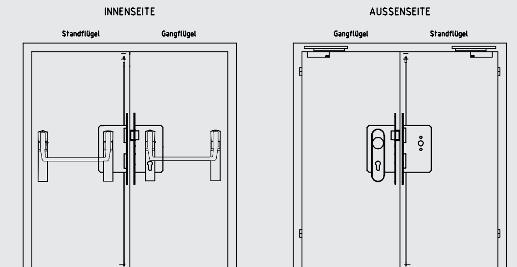
Fluchttürfunktion E
