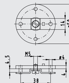
Vorrichtung für Stangenverschluss 3465
