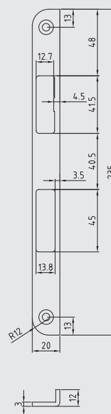
Winkelstulp
