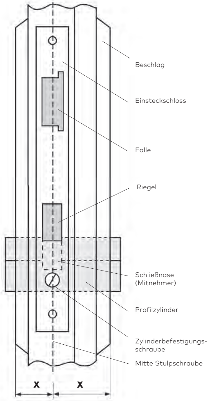
Falztür
