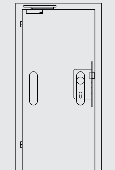
AUSSENSEITE
