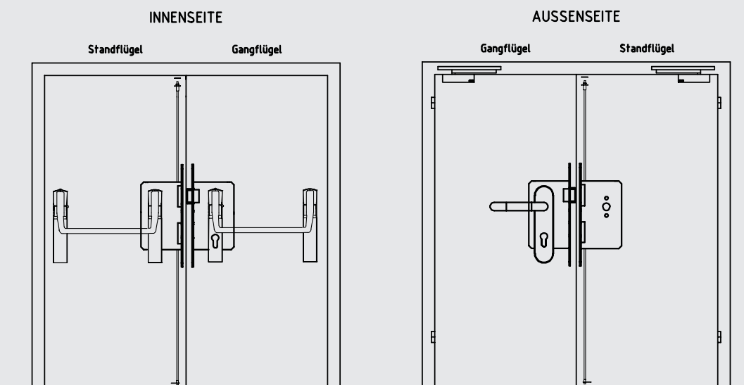
Fluchttürfunktion B
