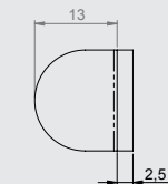
Riegel K/Riegel/83-3-032/AK766
