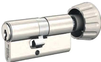
Drehknopf-Kurzzylinder mit rundem Drehknopf (RK)
