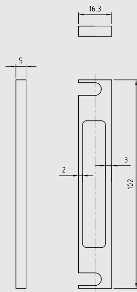
SB/Verstärkung.MV.H/DS
