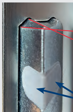
8°-Fallenanzug
