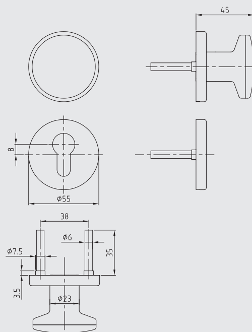
ROSETTEN+KN/PZ/MOD1.3/NR
