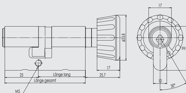
Drehknopf-Kurzzylinder mit rundem Drehknopf (RK)
