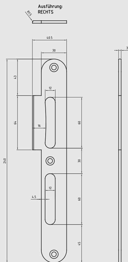
SB/Stumpf.R1,5.RE/NR
