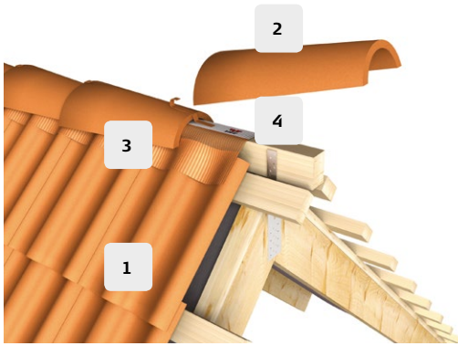
1. IBF tagsten. 2. Rygningssten. 3. Alu-rygningsbånd med ventilation. 4. Rygningsbeslag.
