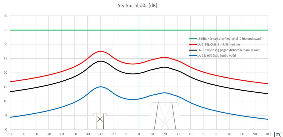
Mynd 18.11 Útreiknaður hávaði þar sem Holtavörðuheiðarlína 3 liggur samsíða stakri byggðalínu (valkostir D að stórum hluta).
