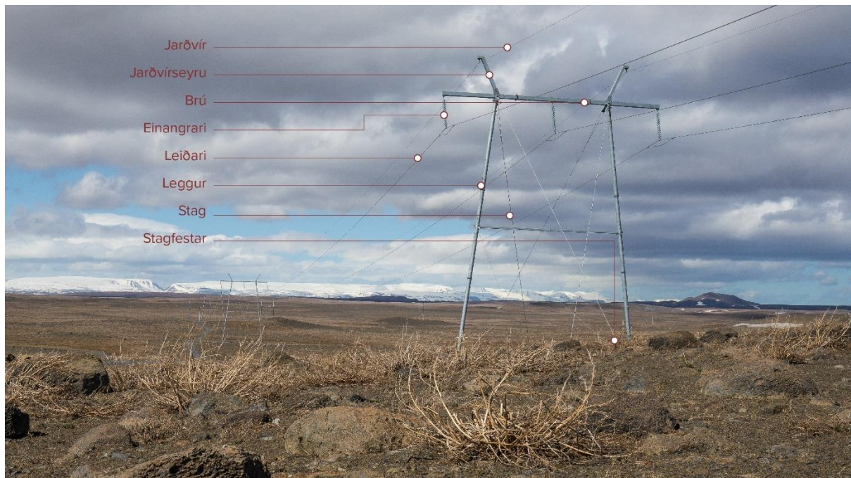
Mynd 6.1 Mastursgerð sem fyrirhugað er að nota næst endum Holtavörðuheiðarlínu 3. Mynd sýnir mastur með jarðvírseyrnum.
