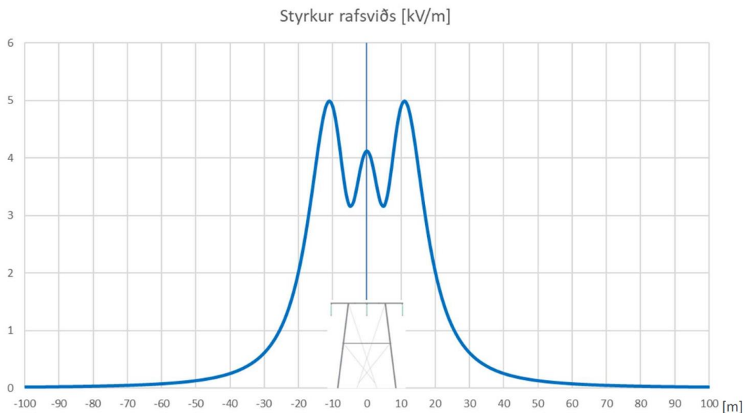
Mynd 18.4 Þversnið rafsviðs í línugötu þar sem HOLTAVÖRÐUHEIDARLÍNA 3 liggur ein (valkostir A og B).
