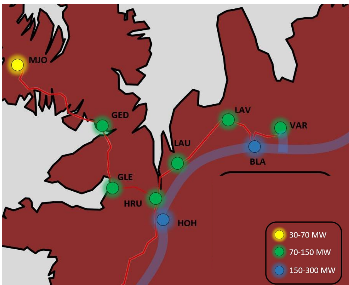
Mynd 22.2 Tiltæk afhendingargeta í flutningskerfi Landsnets á Norðurlandi vestra þegar byggingu nýs byggðalínurings milli Akureyrar og Hvalfjarðar er lokið.
