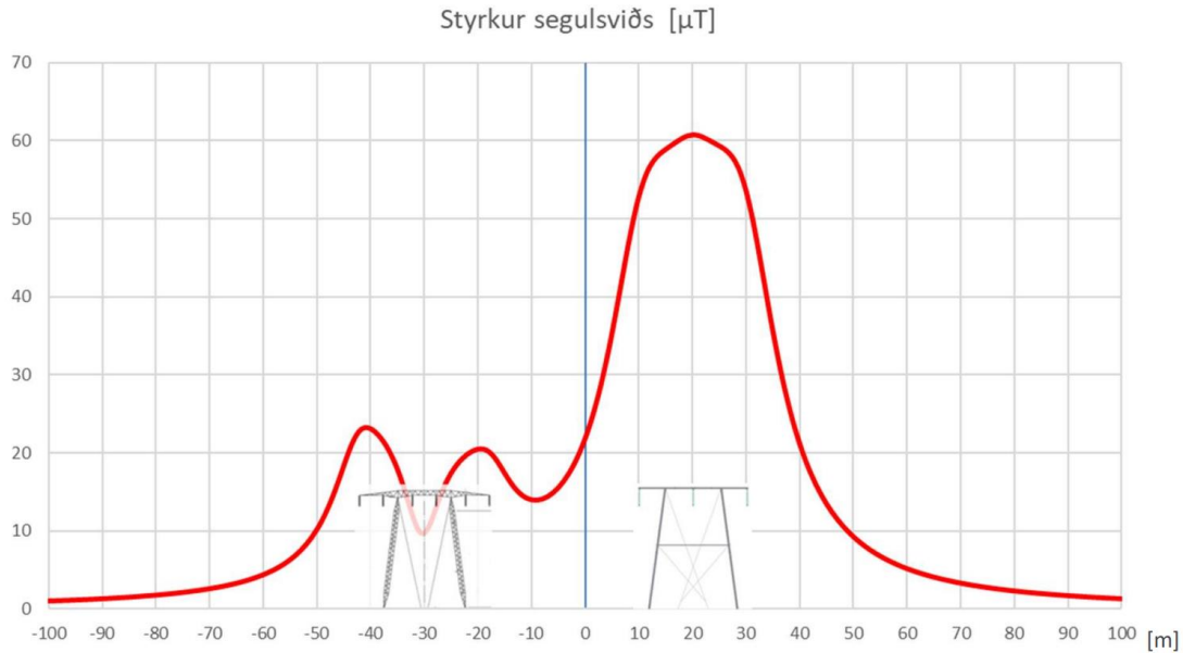
Mynd 18.9 Þversnið segulsviðs í línugötu þar sem Holtavörðuheidarlína 3 liggur samsíða tveimur byggðalínum (valkostir D næst Blönduvirkjun).
