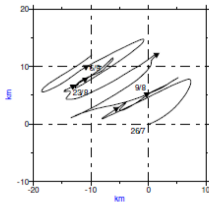
28. mynd. Framskreiddur straumvektor fyrir 8 metra dýpi á lögn C.
