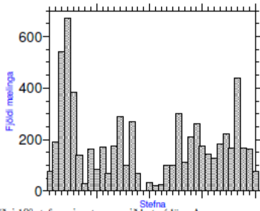
11. mynd. Tíðni 10^\circ stefnugeira straums við botn á lögn A.
