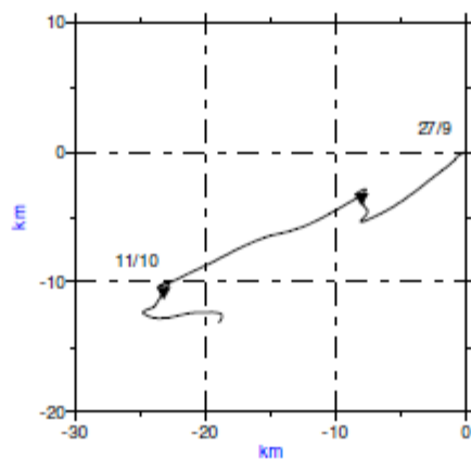
32. mynd Framskreiður straumvektor fyrir 38 metra dýpi á lögn C.
