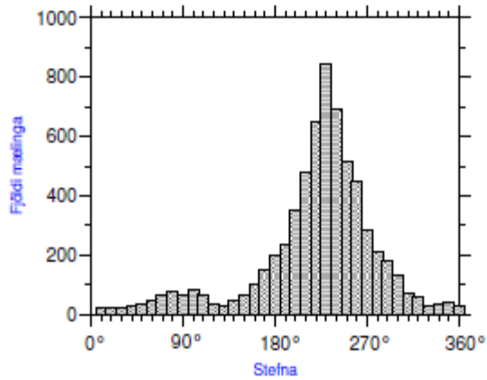
7. mynd. Tíðni 10° stefnugeira á 32 metra dýpi á lögn A.
