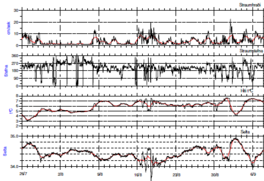
6. mynd. Straumhraði, straumstefna, hitastig og selta frá mælingu á dreifistraumi undir Háubökkum frá 26. júlí til 8. september 2002. Sléttuðu línurnar sýnir 25 tíma keðjumeðaltöl.
