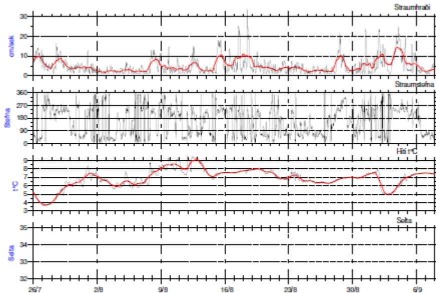
2. mynd. Straumhraði, straumstefna og hitastig frá yfirborðsmælingu undir Háubökkum frá 25. júlí til 8. ágúst 2002. Stéttuðu línurnar sýnir 25 tíma keðjumeðaltöl.
