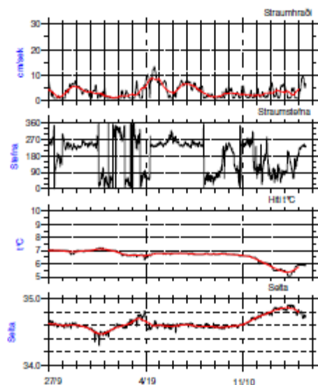
30. mynd. Straumhraði, straumstefna, hitastig og selta frá mælingu á dreiflstraumi á Selstaðavík frá 26. september til 15. október 2002. Sléttuðu línurnar sýna 25 tíma keðjumeðaltöl.
