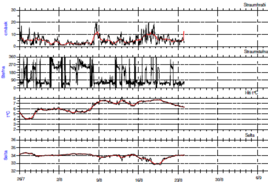
14. mynd. Straumhraði, straumstefna og hitastig og selta frá yfirborðsmælingu á Sörlastaðavík 26. júlí til 24. ágúst 2002. Sléttuðu línurnar sýna 25 tíma keðjumæðaltöl.
