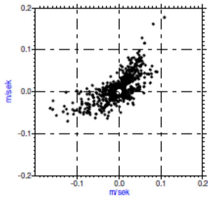
13. mynd Dreifing A-V og N-S straumvektora við botn á lögn A.
