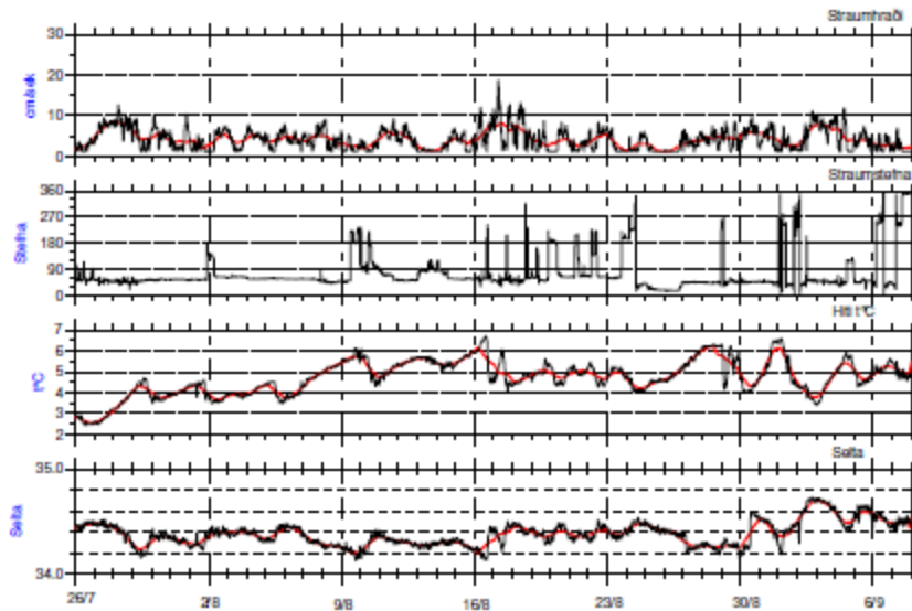
22. mynd. Straumhraði, straumstefna, hitastig og selta frá mælingu við botn á Sörlastaðavík 26. júlí til 8. september 2002. Sléttuðu línurnar sýna 25 tíma keðjumeðaltöl.
