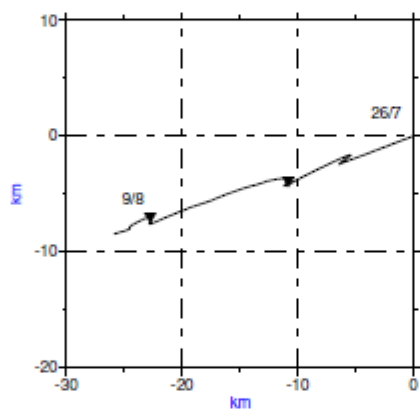
36. mynd. Framskreiður straumvektor fyrir 58 metra dýpi á lögn C.
