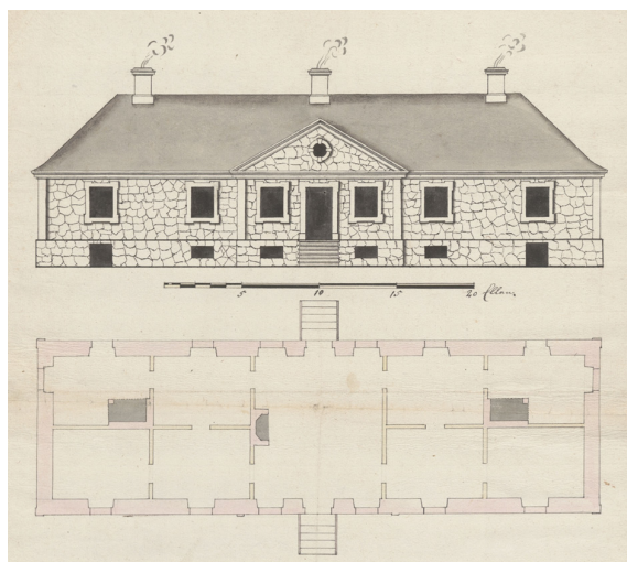
Teikning af húsi amtmanns og stiftamtmanns á Bessastöðum gerð vegna ýmissa viðgerða á því árið 1736.
