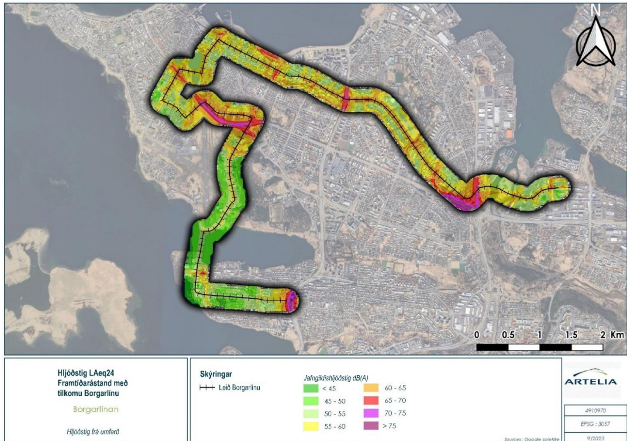
Mynd 7.13 24 klst. jafngildishljóðstig ( L_{Aeq24} ) m.v. framtíðartilvik með Borgarlínunni (árið 2027).
