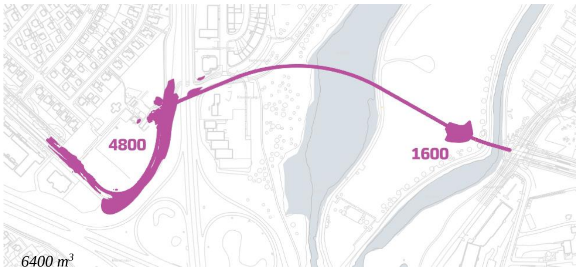
Mynd 7.31 Áætlaður gröftur og skeringar vegna brúar yfir Elliðaár (mynd er ekki í skala).
