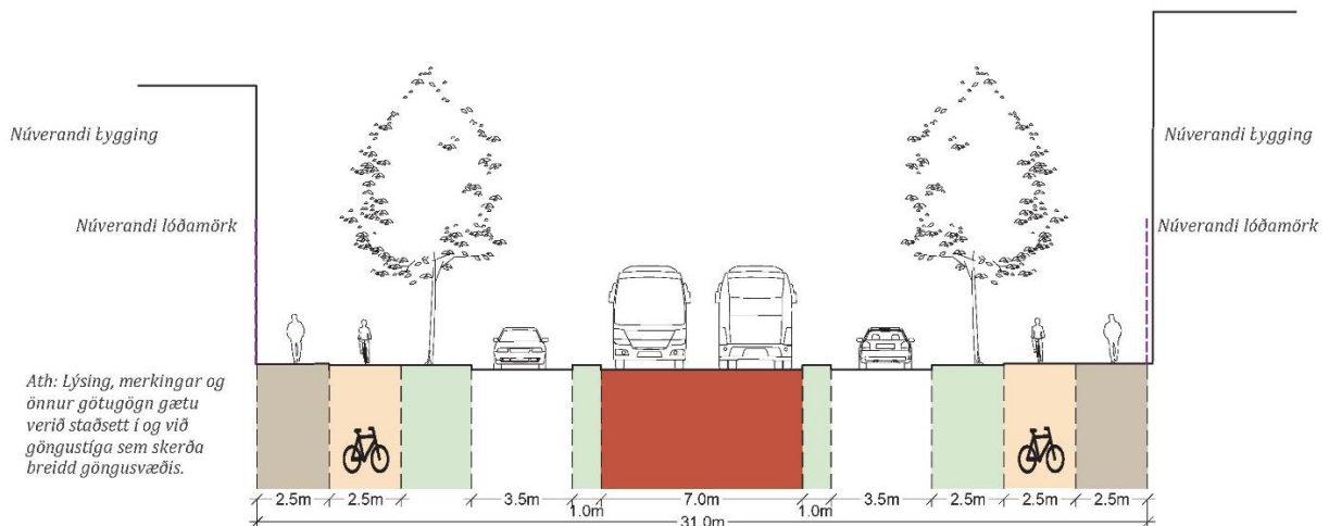
Mynd 5.37 Þversnið af göturými við Arnarhlíð, suður af gatnamótum við Valshlíð 41 , horft til suðurs.
