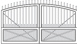
Arch 6'H x 12'W
