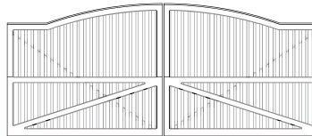
Annisquam Arch 6'H x 16'W
