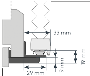
Schnitt Klemmklebeträger
