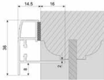
Schnitt Fensterflügel mit Rahmenprofil M8R
