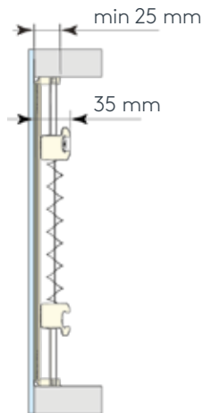
Schnitt Klebeleiste
