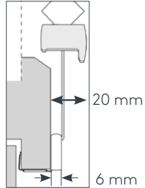
Schnitt Klemmträger
