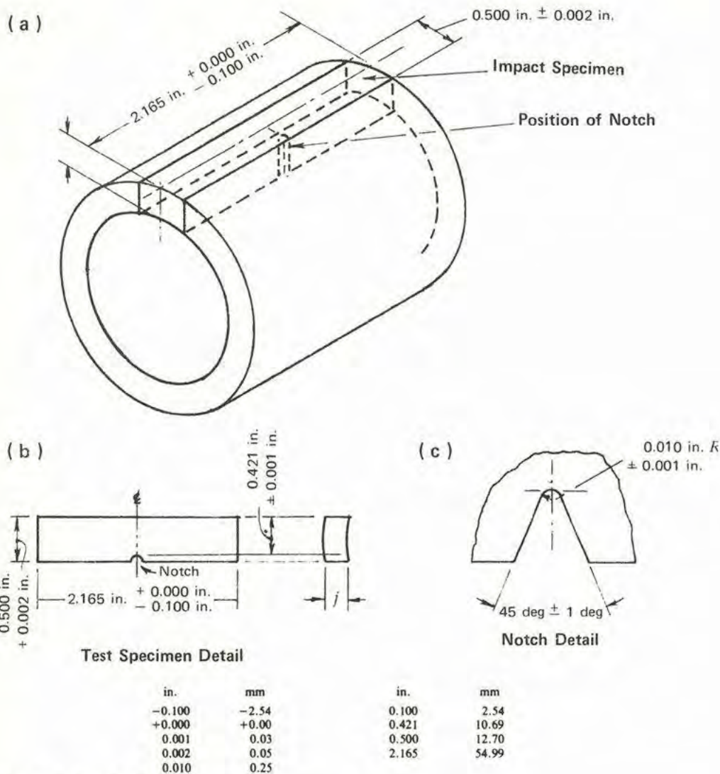
FIG. 2 Impact Test Specimen.
