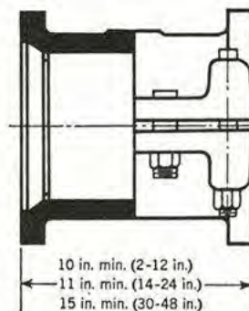
Fig. 10.11. Mechanical-Joint Split Sleeves
