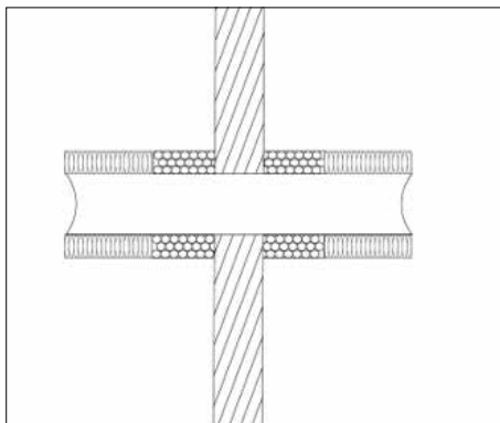
Fig. 5: Viser en (Local Interrupted (LI)) rørisolering, der går ud på hver side af konstruktionen, med det minimum angivne antal mm på hver side.
