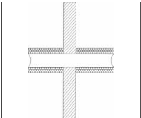
Fig. 4: Viser en Continued Interrupted (CI) rørisolering - rørisoleringen afbrydes og går ikke med gennem konstruktionen.
