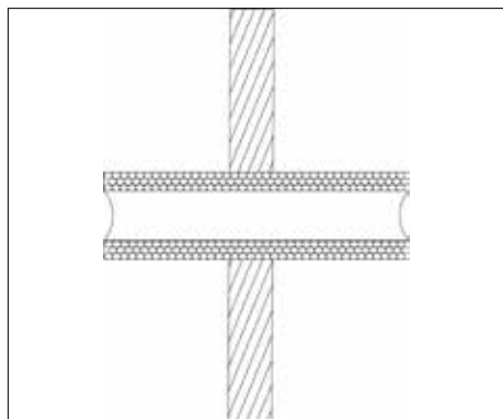
Fig. 1: Viser en Continued Sustained (CS) rørisolering, hvor isoleringen føres med gennem konstruktionen i hele rørets længde*.
