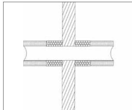
Fig. 6: Viser en Continued Interrupted (CI) løsning, hvor isoleringen ikke er ført med gennem konstruktionen og den øvrige del af røret er isoleret med isoleringstype, der ikke nødvendigvis har indflydelse på den testede brandluknings forudsætninger.
