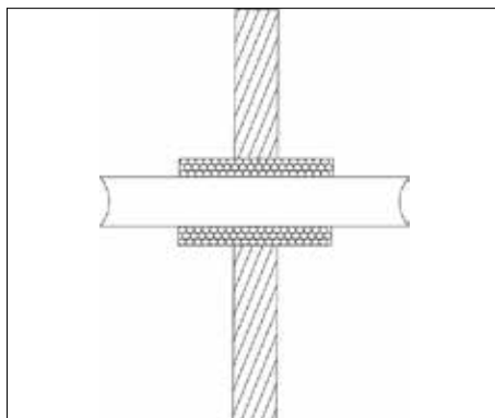
Fig. 2: Viser en Local Sustained (LS) løsning, hvor isoleringen kun føres med gennem konstruktion, med et givent antal mm ud på hver side*.
