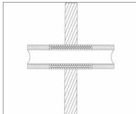
Fig. 3: Viser en Local Sustained (LS) rørisolering - isoleringen er ført med gennem konstruktionen. Den øvrige del af røret er isoleret med en isoleringstype, der ikke nødvendigvis har indflydelse på den testede brandluknings forudsætninger.
