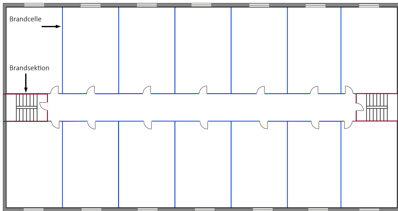
Eksempel på opdeling af plan i brandceller og brandsektioner.
