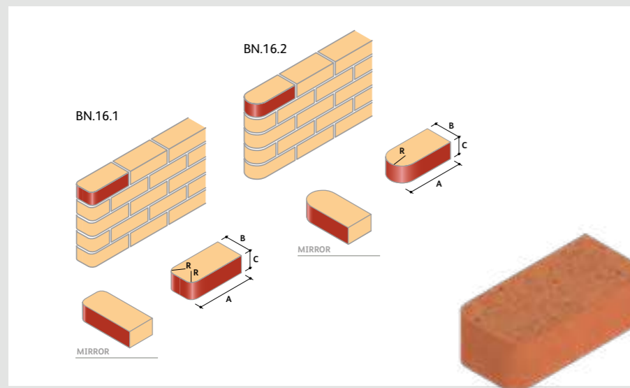
BN.16 Cownose
