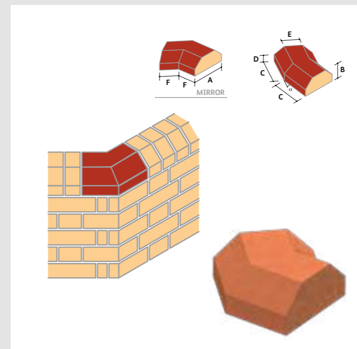
AN.18 Double Cant Angle
