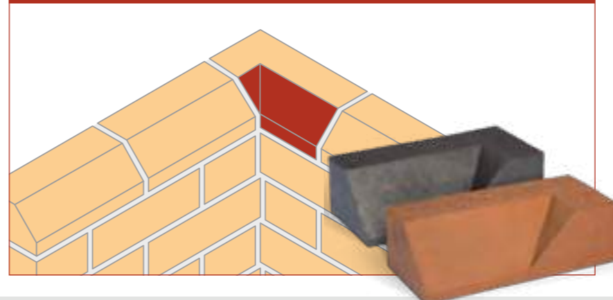
PL.4.1/PL.4.2 Plinth Internal Return
