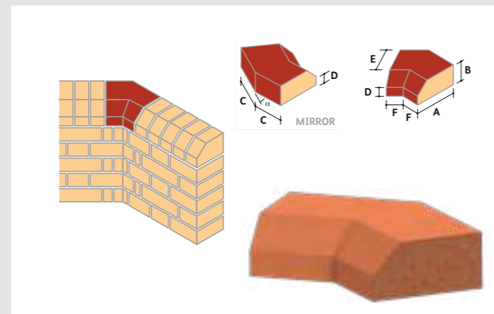
AN.11 Single Cant Internal Angle
