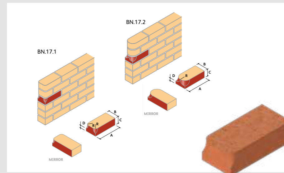
BN.17 Cownose Stop
