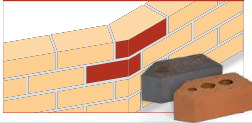
AN.1.2 45° Squint Brick
