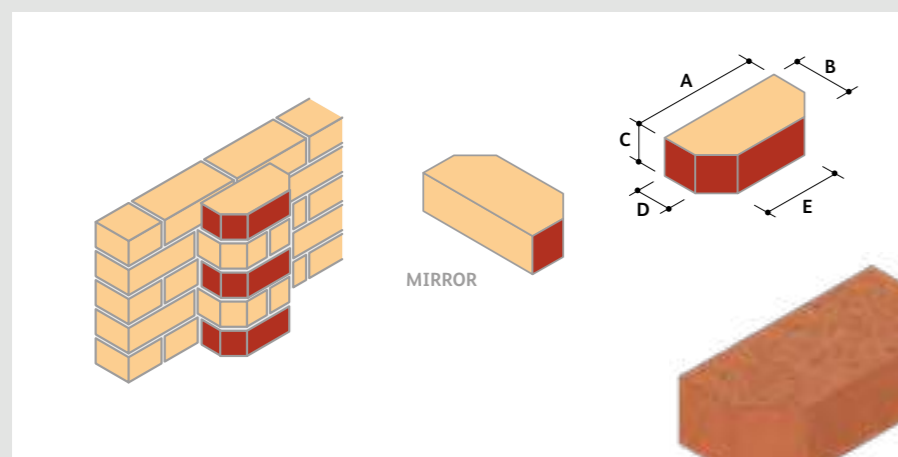
AN.6 Double Cant
