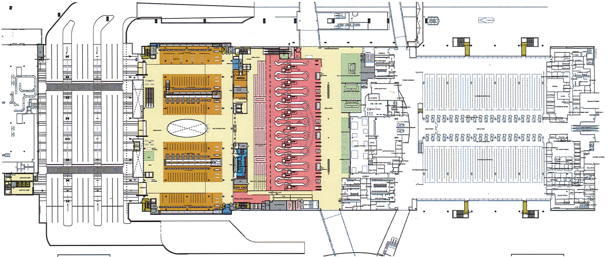
1 FIS_L2 DEPARTURES LEVEL - CD 03.JUL.18 AR - 105 SCALE: 1" = 40'-0"
