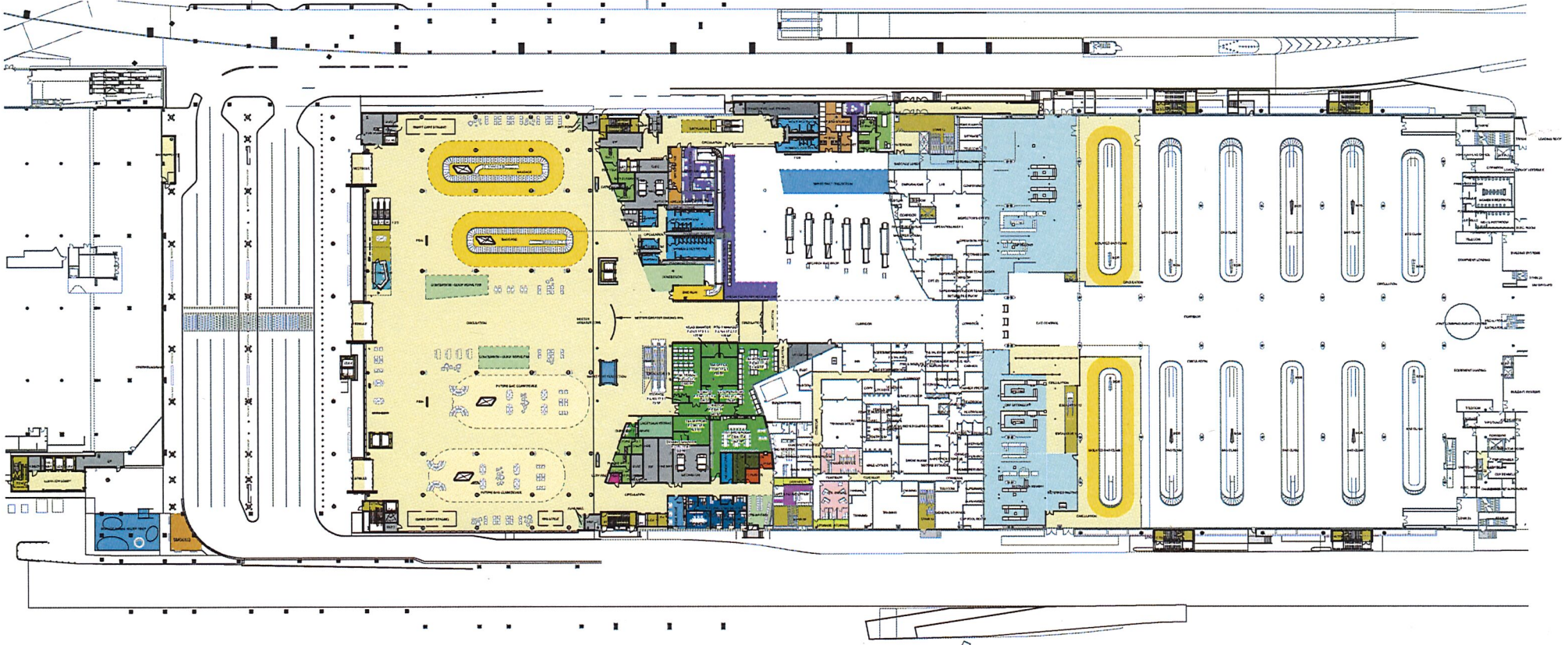
1 FIS_L1 ARRIVALS LEVEL - CD - Phase 1 00 JEA AR - 103.1 SCALE: 1" = 40'-0"
