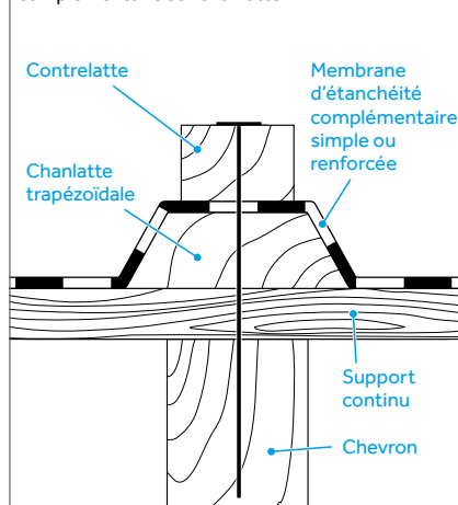
Figure 1 : mise en œuvre de l'étanchéité complémentaire sur chanlatte
