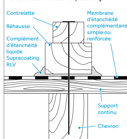
Figure 2 : mise en œuvre de l'étanchéité complémentaire sous réhausse + Supracoating RLV
