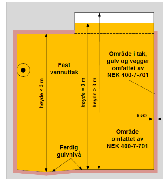
Figur 701B – Område dekket av 701, sett fra siden
