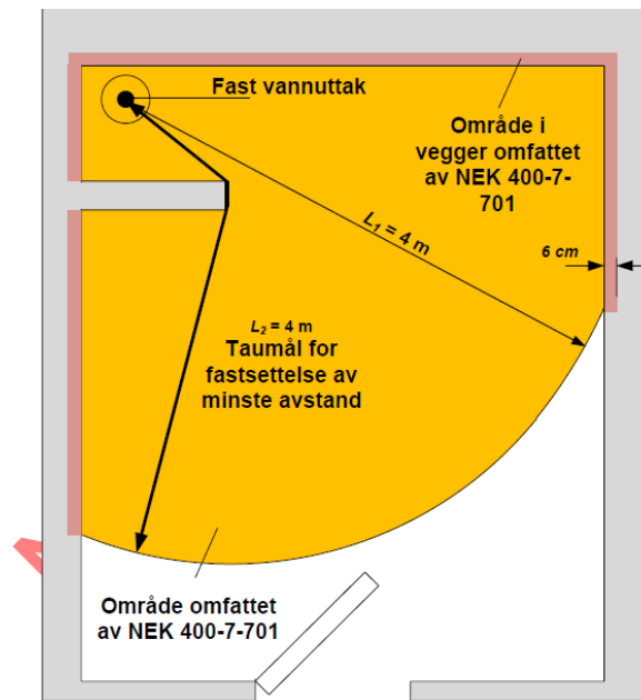
Figur 701A – Område dekket av 701, sett ovenfra
