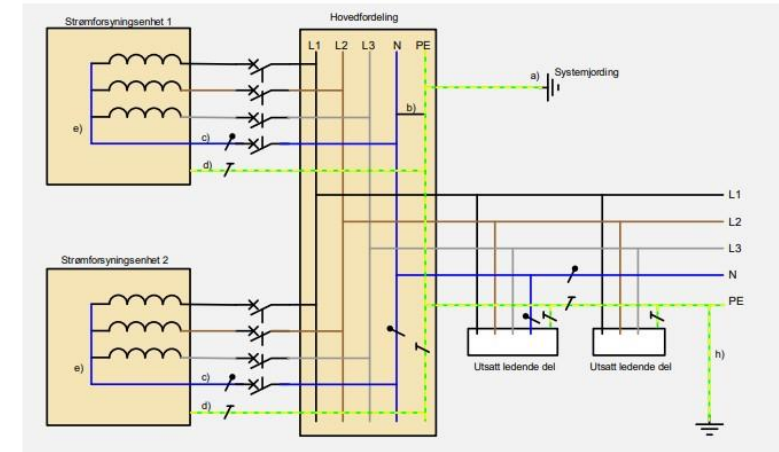
Figur 1: TN system (TN-S system) med kun interne strømforsyningsenheter, prinsippskisse
