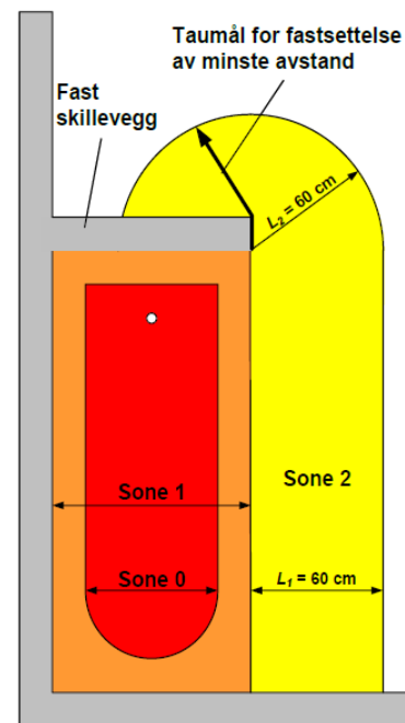
Figur 701F - Eksempel på soner for et badekar, med en avdeling, sett ovenfra
