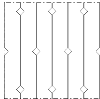
PANELDETALJERING – TYPDETALJ SKALA 1:20
