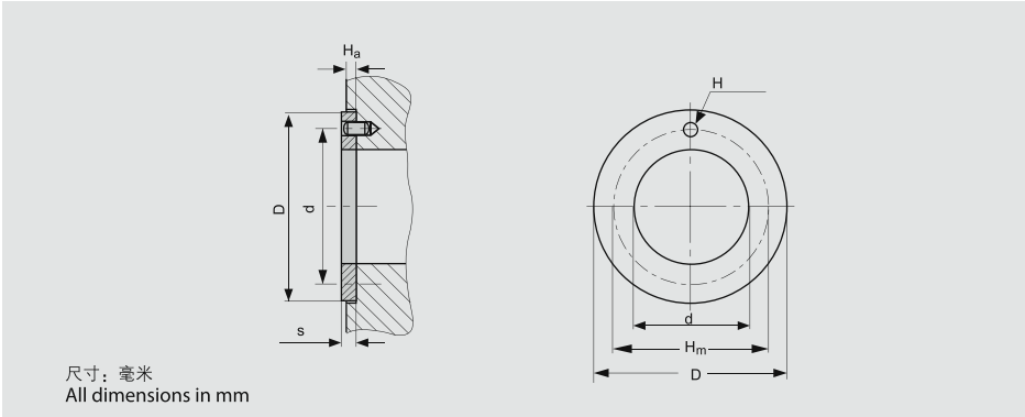
垫片型号标注方式 Washer Symbol
