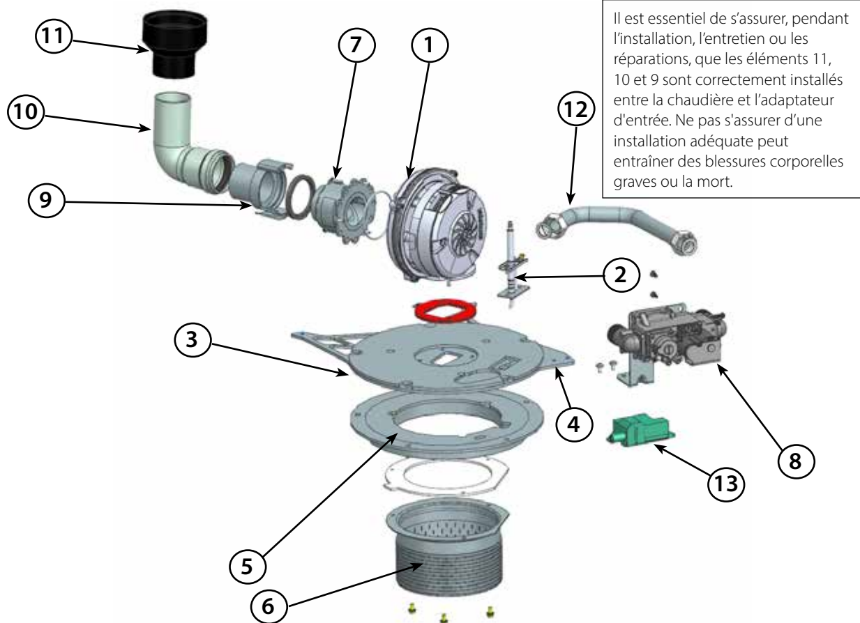
Fig. 42 - Composants du brûleur de l'appareil Instinct FSB Solo/Combi 155
