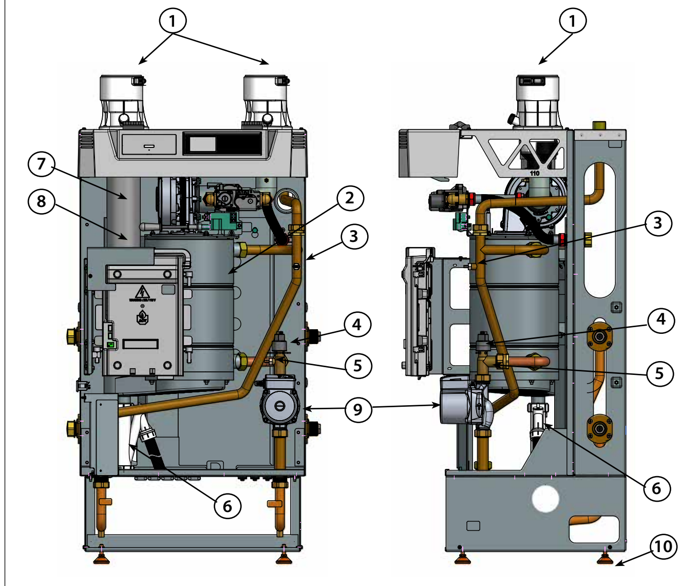
Fig. 36 - Composants internes de l'appareil Instinct FSB Solo 110
