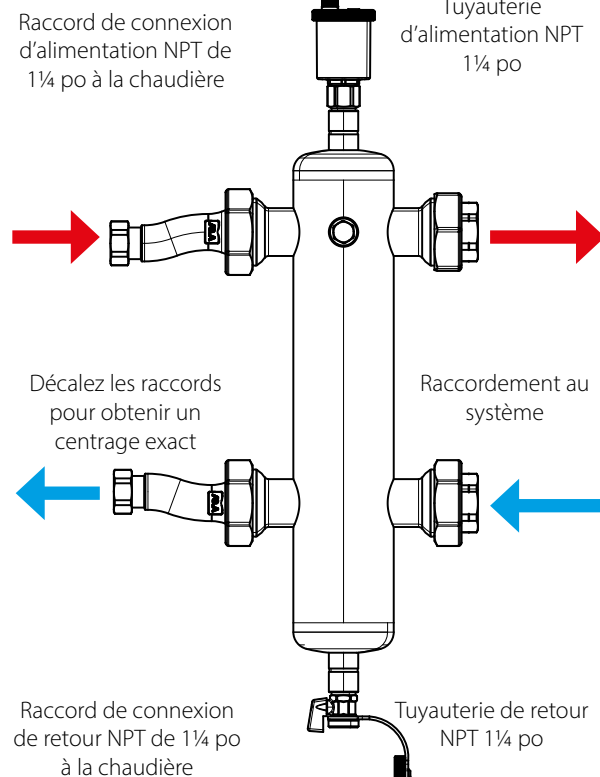
Fig. 12 - Séparateur hydraulique de 1 1/4 po utilisé sur les modèles 199
