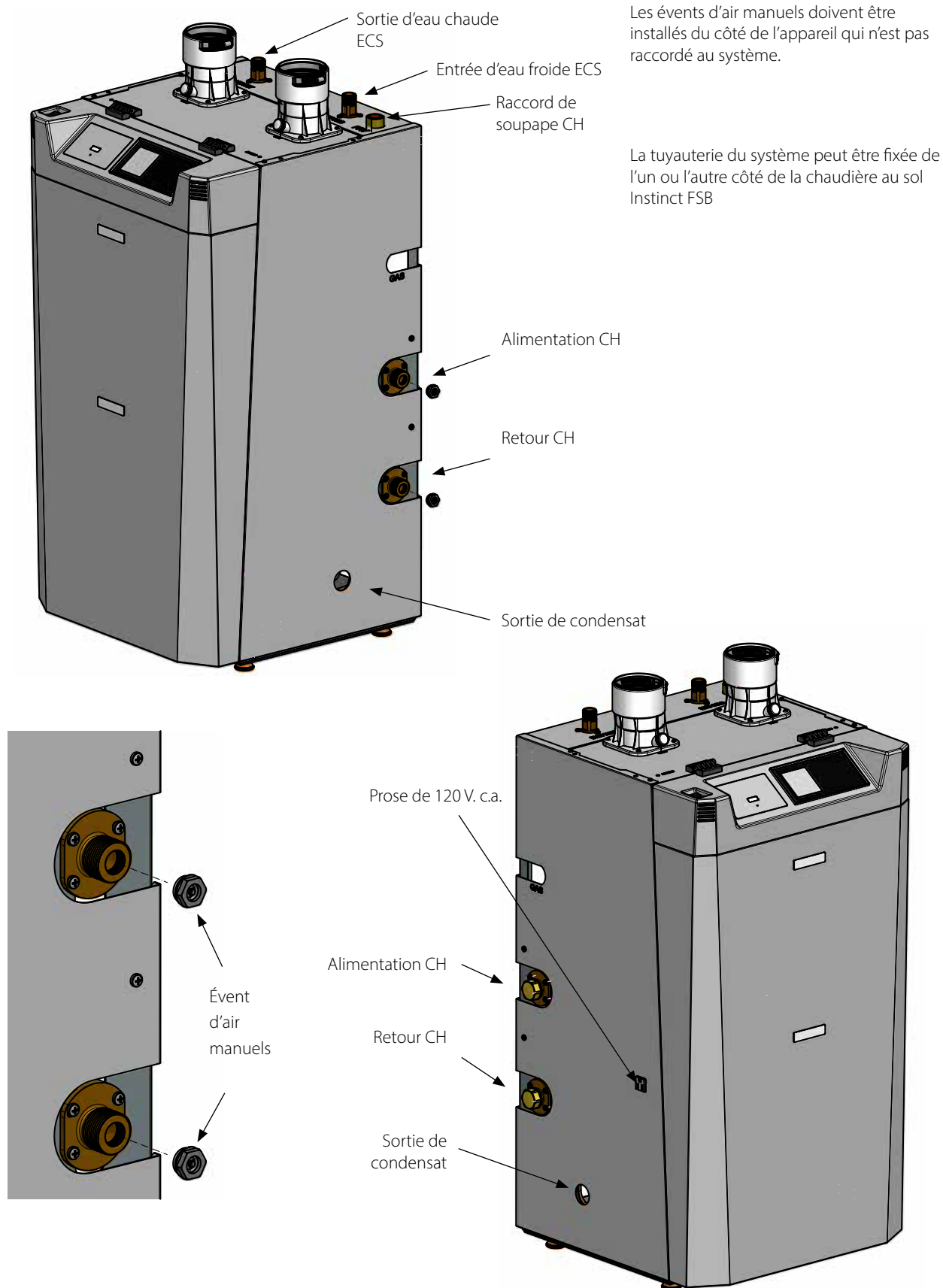
Fig. 10 - Évent d'air Instinct FSB - Vue éclatée
