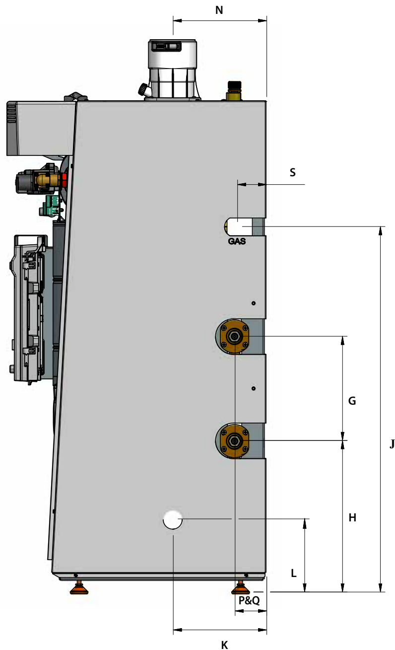
Fig. 53 - Vue du côté droit Instinct FSB Combi 155
