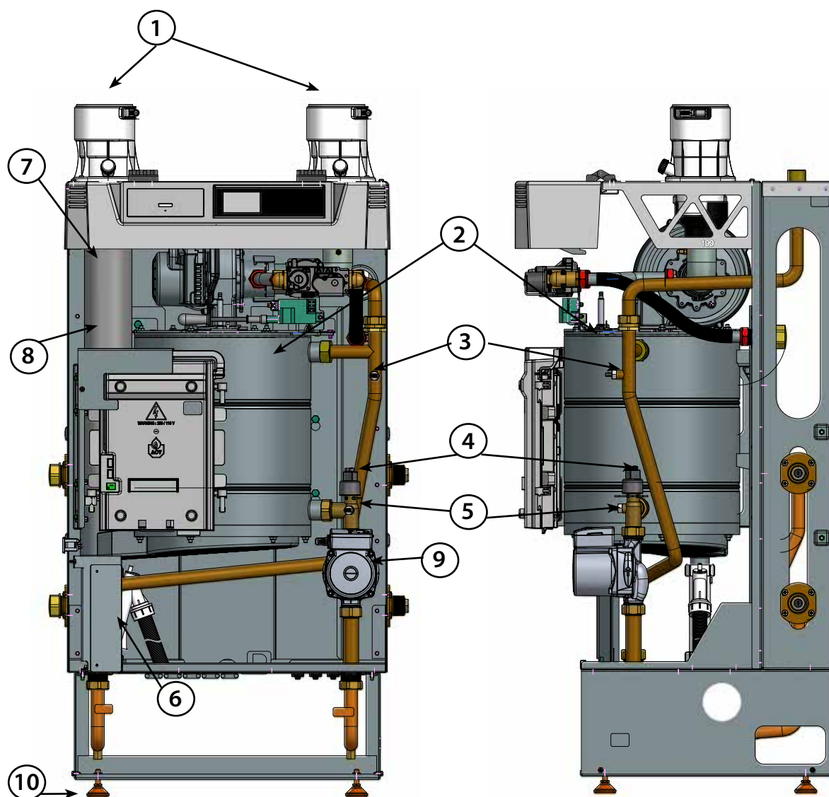
Fig. 39 - Composants internes de l'appareil Instinct FSB Solo 199
