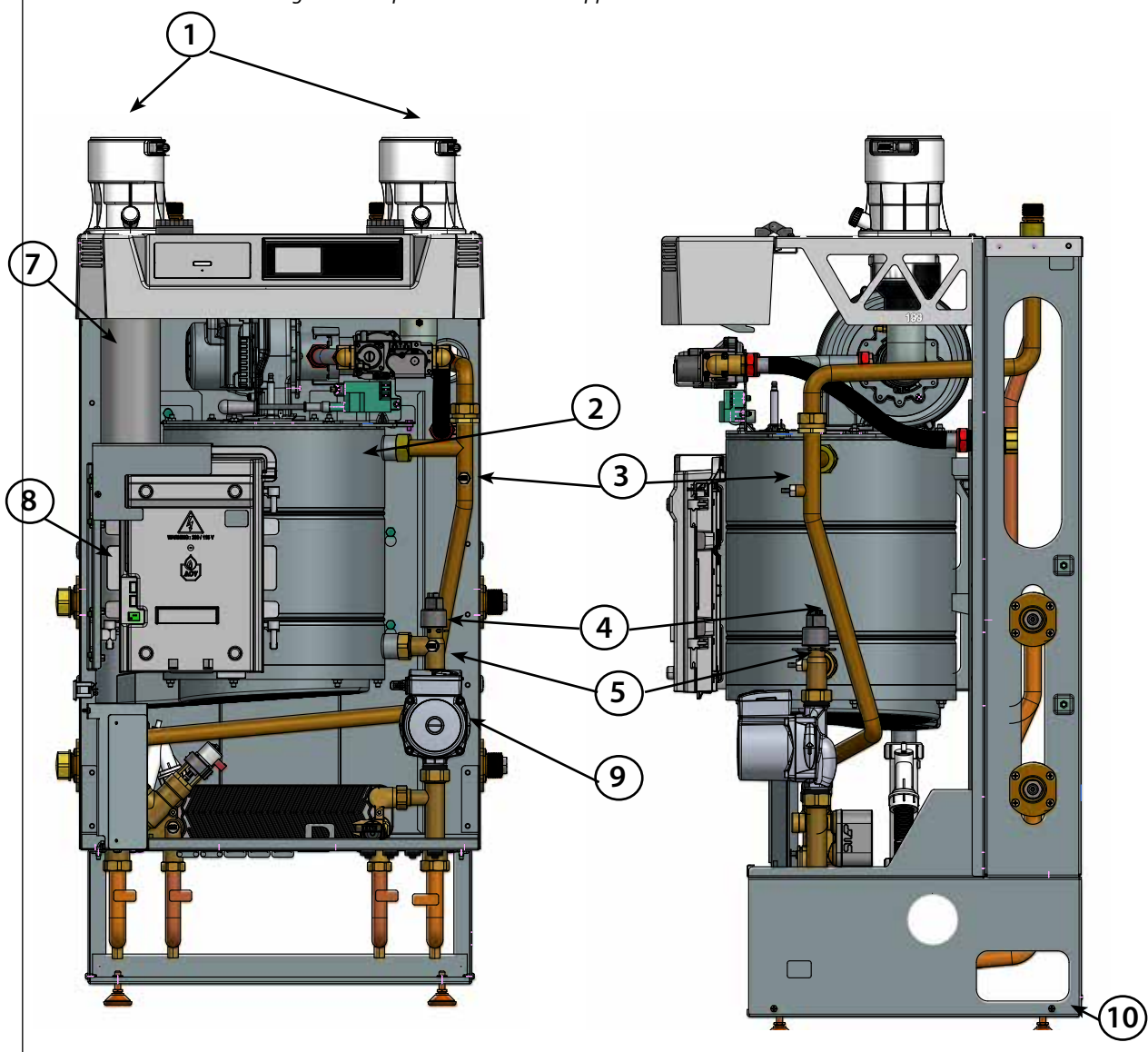
Fig. 40 - Composants internes de l'appareil Instinct FSB Combi 199
