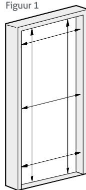
Kozijnopening opmeten
