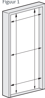
Kozijnopening opmeten
