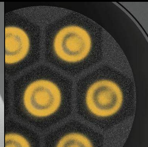
Homogenisierende Streuscheiben verhindern unerwünschte Effekte wie Abrisskanten des Lichts.
