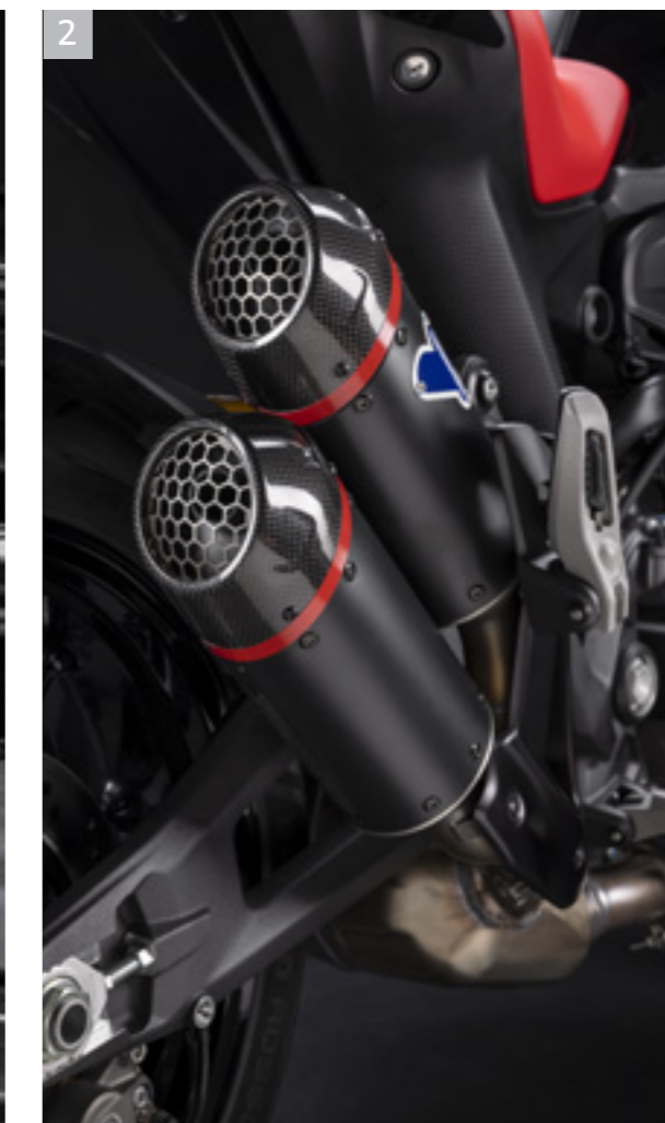
2 Pre-silenziatore e doppio terminale Termignoni omologato, catalizzatore e 2 sonde lambda
