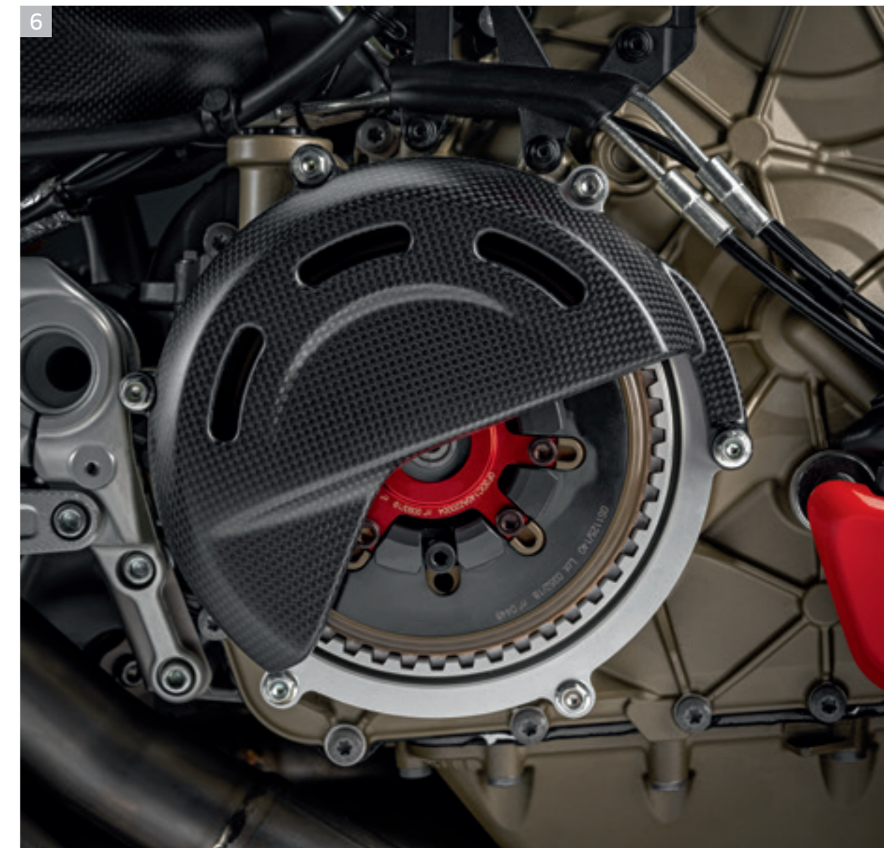
6 Kit frizione a secco. Cover frizione a secco in carbonio.
